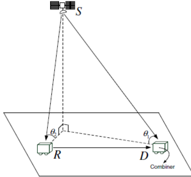
Σχήμα 4.1: Η γεωμετρική διάταξη του θεωρούμενου συνεργατικού συστήματος με ένα αναγεννητικό επαναλήπτη [32].
