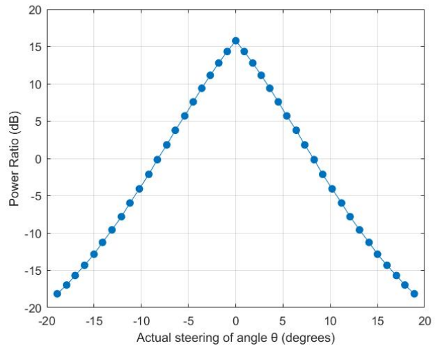
Σχήμα 4.38: Διάγραμμα συσχέτισης ισχύος (Power Ratio) μεταξύ κύριου λοβού και πρώτου grating lobe, (4 AEs, 5μm pitch).
