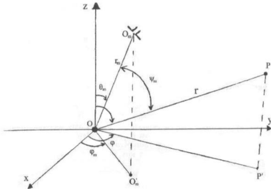
Σχήμα 2.5 Σύστημα συντεταγμένων για την ανάλυση στοιχειοκεραιών [29].
