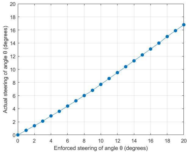
Σχήμα 4.10: Διάγραμμα απόκλισης γωνίας επιβαλλόμενης στροφής στη διεύθυνση του κύριου λοβού, (2 AEs, 6μμ pitch).
