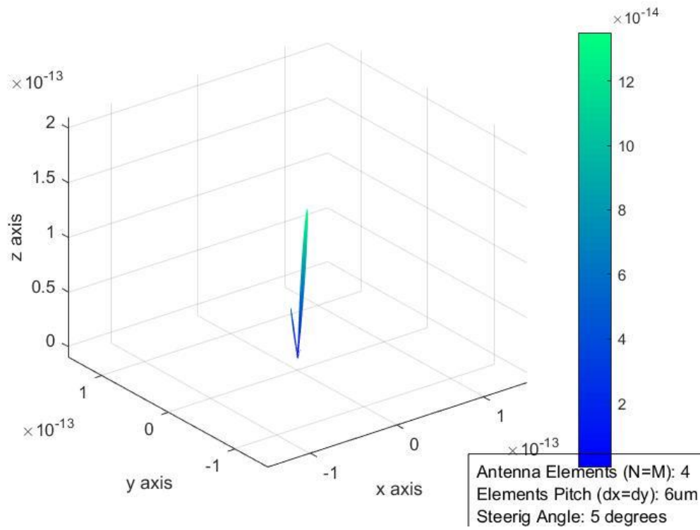
Σχήμα 3.20: Τρισδιάστατο διάγραμμα ακτινοβολίας της έντασης της επίπεδης οπτικής στοιχειοκεραίας, αποτελούμενης από 4 στοιχεία με απόσταση 6μm και στα δύο επίπεδα και στροφή 5 ο στην διεύθυνση του κύριου λοβού στο αζιμουθιακό επίπεδο.
