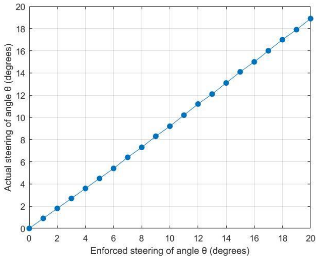
Σχήμα 4.35: Διάγραμμα απόκλισης γωνίας επιβαλλόμενης στροφής στη διεύθυνση του κύριου λοβού, (4 AEs, 5μm pitch).
