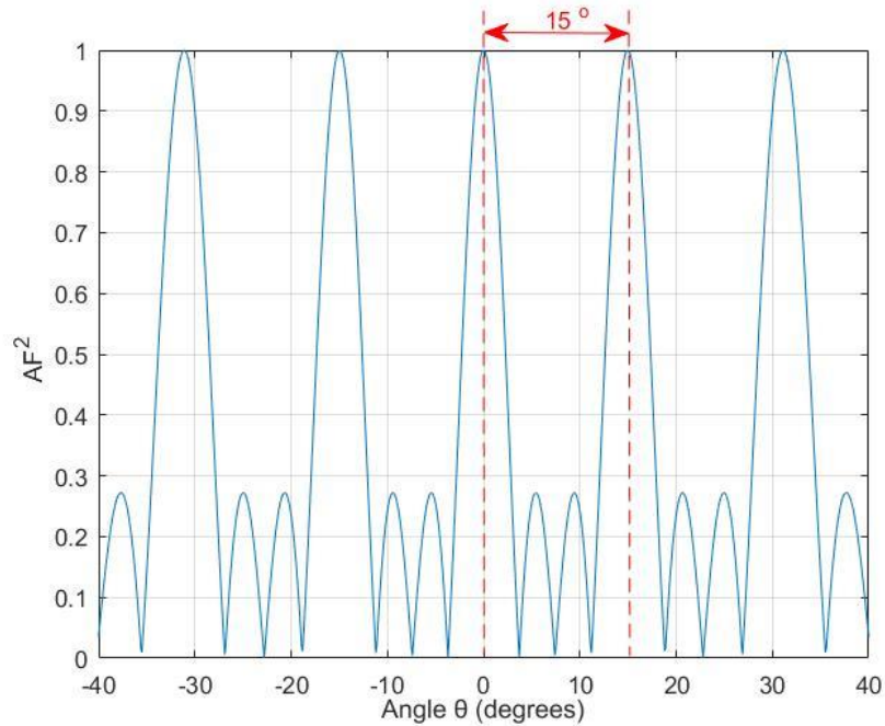
Σχήμα 3.13: Παράγοντας διάταξης που αντιστοιχεί σε γραμμική στοιχειοκεραία 4 στοιχείων με απόσταση 6μm και γωνία στροφής \theta^\circ .
