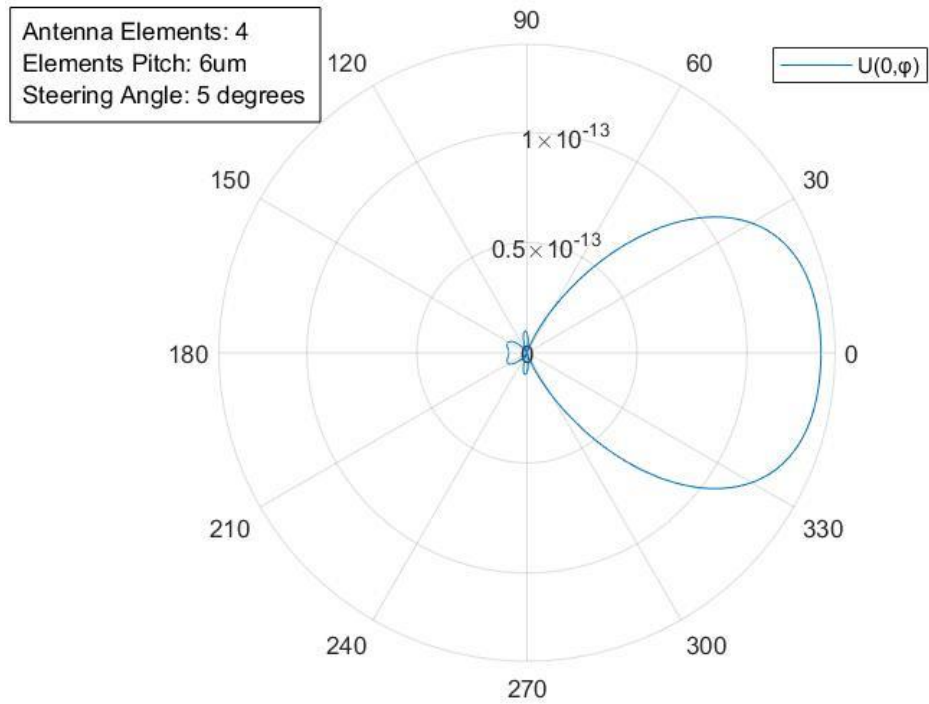
Σχήμα 3.15 Πολικό διάγραμμα ακτινοβολίας της έντασης της στοιχειοκεραίας, αποτελούμενης από 4 στοιχεία με απόσταση 6mm, για σταθερή γωνία ανώμωσης ( \theta = 0^\circ ). Στην περίπτωση αυτή έχει πραγματοποιηθεί στροφή 5^\circ στην διεύθυνση του κύριου λοβού.
