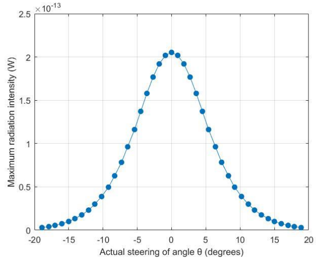
Σχήμα 4.36: Διάγραμμα απόλειας της μέγιστης έντασης ακτινοβολίας του κύριου λοβού, (4 AEs, 5μm pitch).
