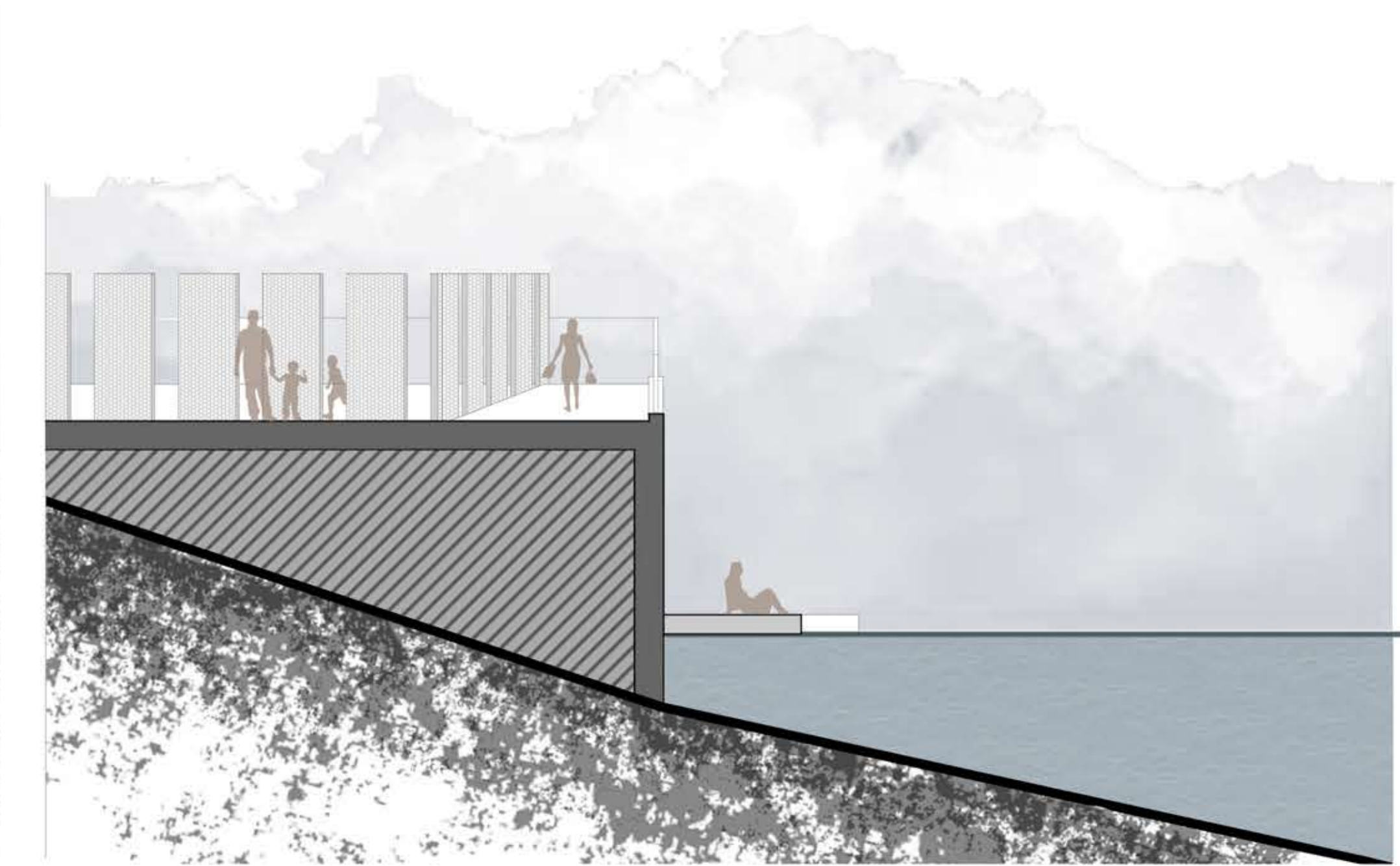
ΤΟΜΗ Δ-Δ
