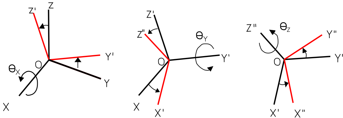
Σχήμα 3.1: Περιστροφή Καρτεσιανού άξονα μέσω των γωνιών Euler \theta_x, \theta_y, \theta_z
