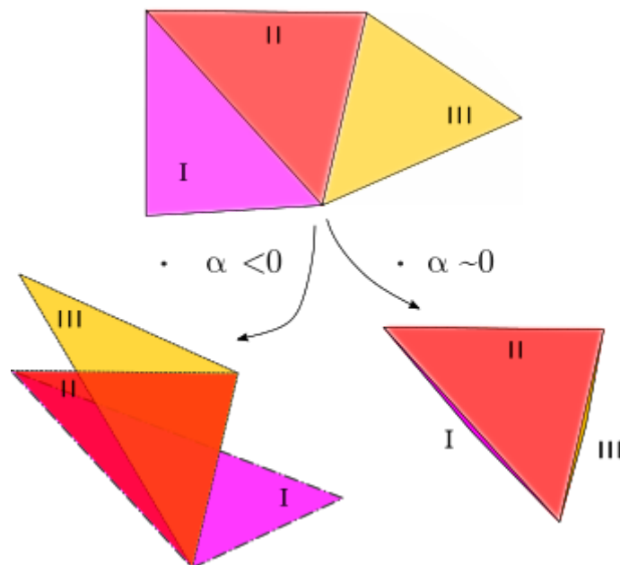
Σχήμα Α.1: Αρχικά τα τρίγωνα I,II,III έχουν \alpha > 0 , μετά από δύο τυχαίες παραμορφώσεις, αριστερά του σχήματος τα τρίγωνα I,III υπολογίζονται με \alpha < 0 ενώ τα τρίγωνα I,III δεξιά υπολογίζονται με \alpha \approx 0
