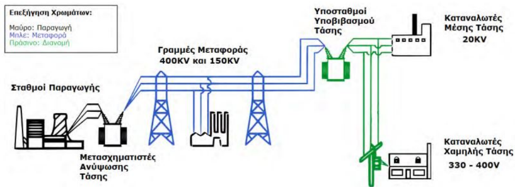
Figure 2.1: Γενική απεικόνιση του ελληνικού ΣΗΕ [2]
