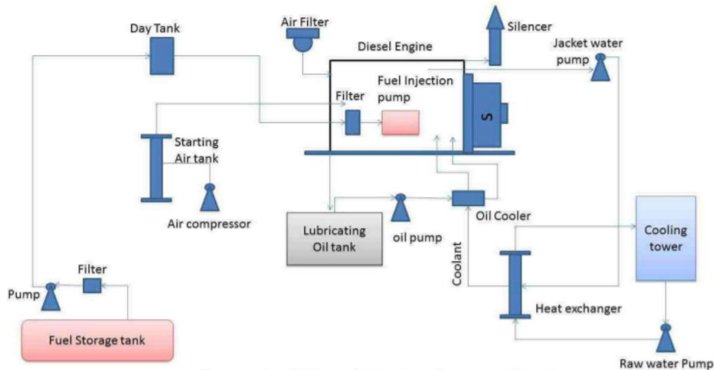
Figure 2.7: Ντιζελοηλεκτρικός σταθμός
