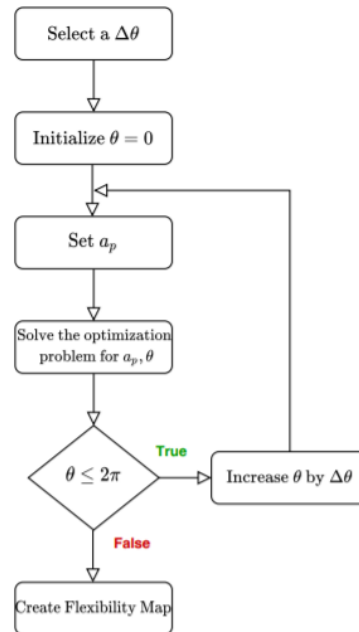
Figure 3.4: Διάγραμμα ροής για την προτεινόμενη μέθοδο [41]
