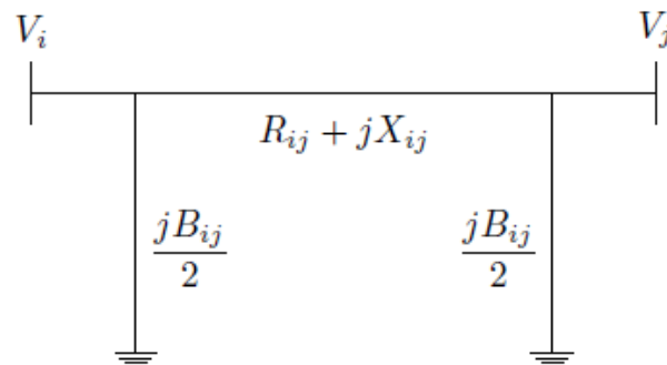
Figure 4.3: \pi -μοντέλο γραμμής μεταφοράς [36]
