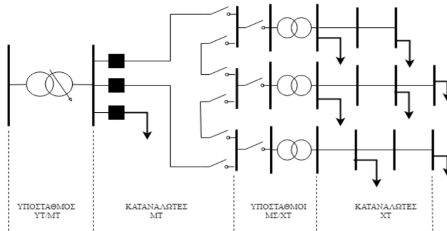
Figure 2.14: Τοπολογία βροχοειδούς δικτύου διανομής
