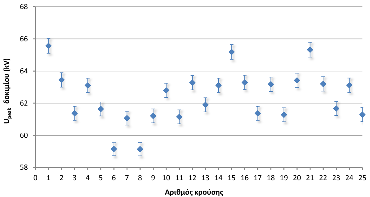
Γράφημα 4.7 Αβεβαιότητα τάσης δοκιμίου Β' 10% υγρασία.
