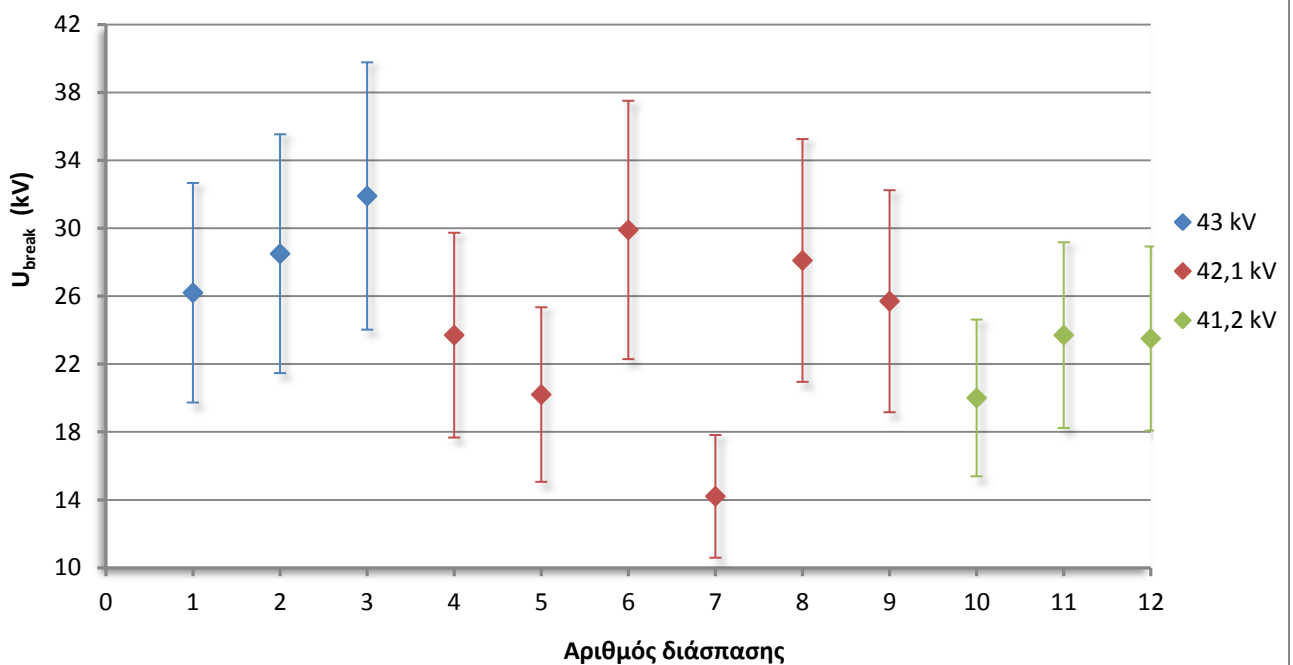
Γράφημα 4.8_Αβεβαιότητα τάσης τη στιγμή της διάσπασης ανά επίπεδο τάσης, για το δοκίμιο Β' 10% υγρασία.
