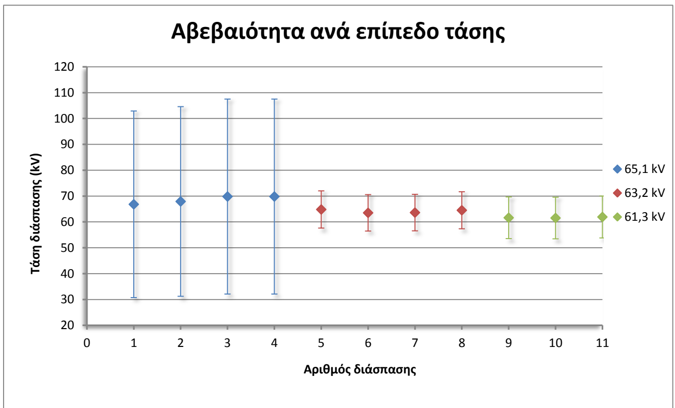
Γράφημα 4.6 Αβεβαιότητα τάσης τη στιγμή της διάσπασης ανά επίπεδο τάσης, για το δοκίμιο Β 5% υγρασία.
