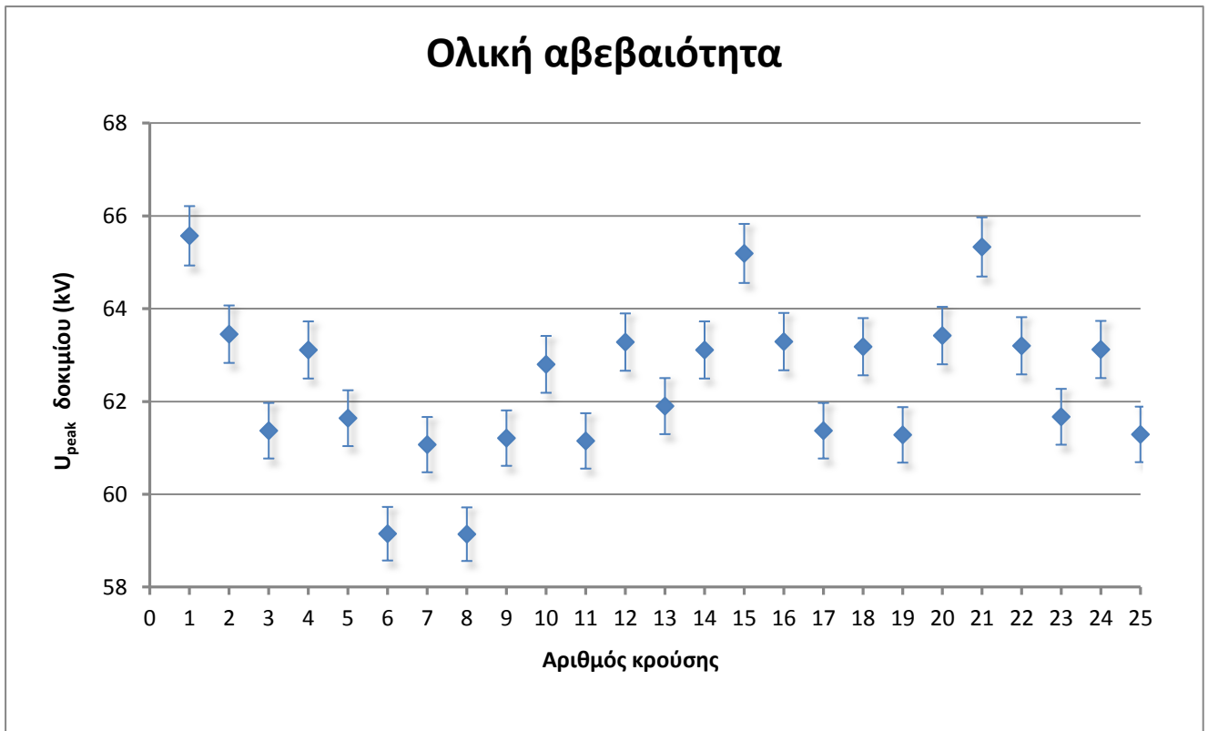
Γράφημα 4.5 Αβεβαιότητα τάσης δοκιμίου Β 5% υγρασία.
