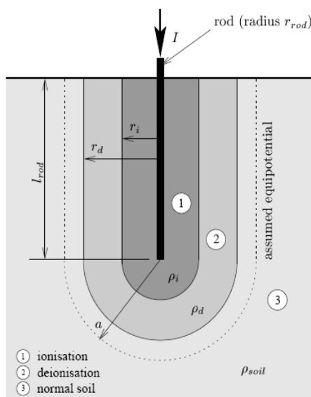
Σχήμα 1.3 Μοντέλο Liew και Darveniza [12].
