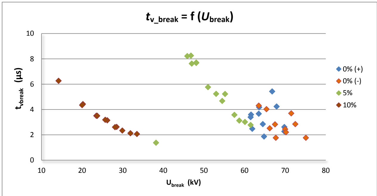
Γράφημα 4.17 Χρόνος διάσπασης συναρτήσει της τάσης διάσπασης για το δοκίμιο Β'.
