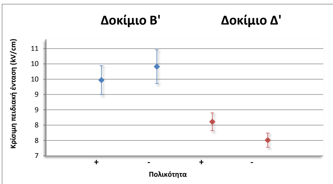
Γράφημα 4.15 Τάση διάσπασης για αρνητική και θετική πολικότητα σε κάθε εδαφικό δείγμα.
