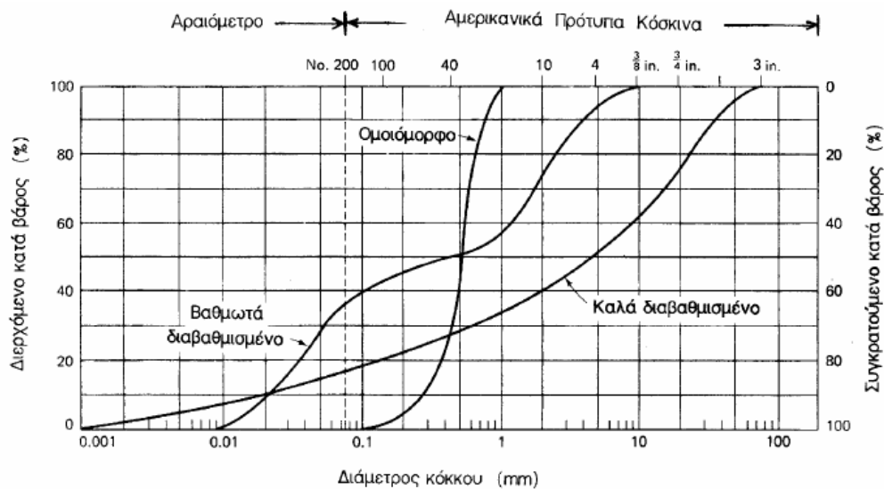
Σχήμα 2.14 Διάγραμμα κοκκομετρικής διαβάθμισης εδαφών.
