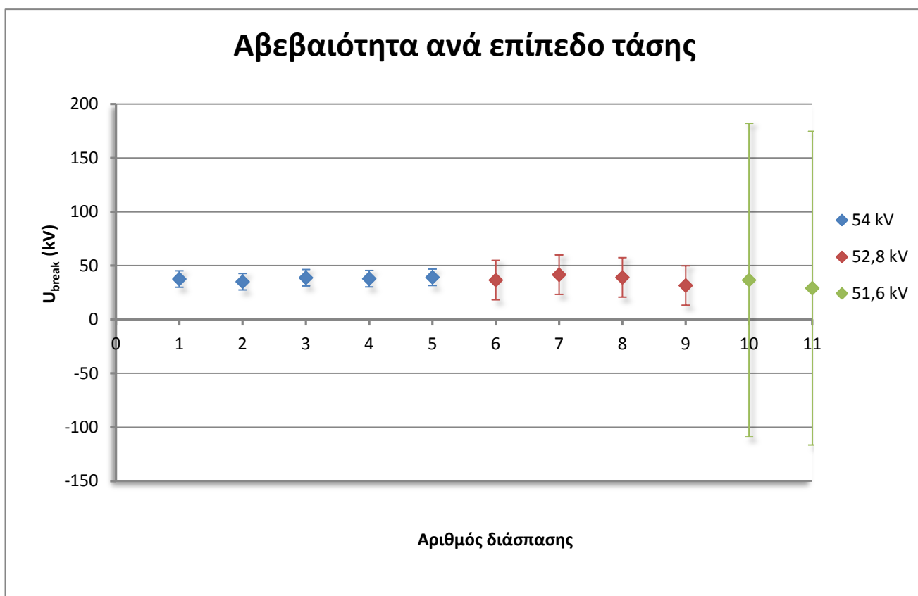
Γράφημα 4.14 Αβεβαιότητα τάσης τη στιγμή της διάσπασης ανά επίπεδο τάσης Δ' 5% υγρασία.
