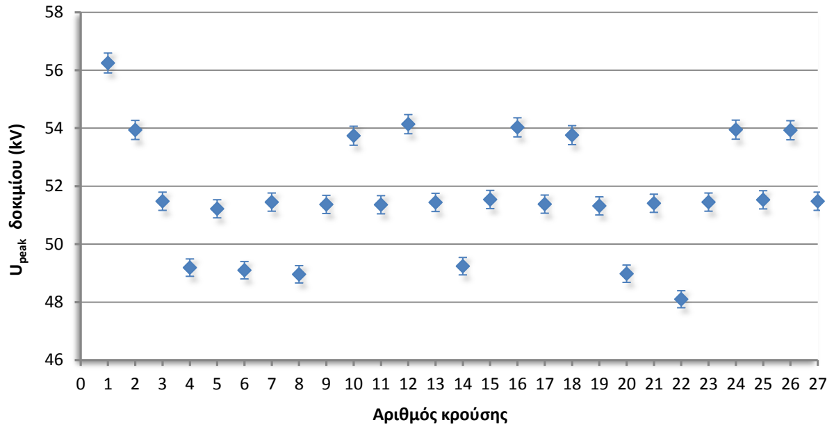
Γράφημα 4.11 Αβεβαιότητα τάσης δοκιμίου Δ' 0% υγρασία, αρνητική πολικότητα.
