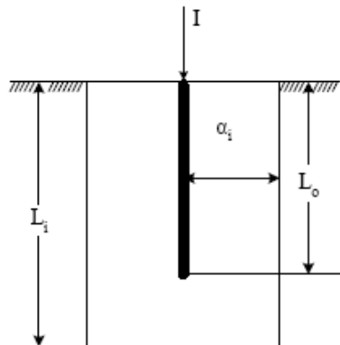
Σχήμα 1.1 Μοντέλο Bellaschi [15].
