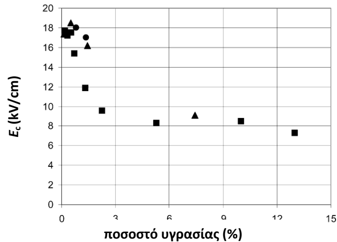
Σχήμα 1.8 Μεταβολή της κρίσιμης έντασης συναρτήσει της περιεκτικότητας του χώματος σε υγρασία.
