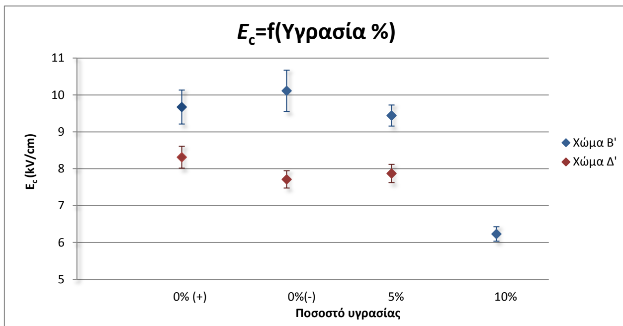
Γράφημα 4.16 Κρίσιμη πεδιακή ένταση και αβεβαιότητα για κάθε επίπεδο ποσοστού υγρασίας των δυο εδαφικών δειγμάτων.
