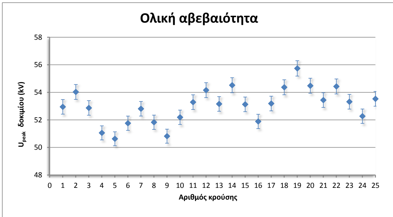
Γράφημα 4.13 Αβεβαιότητα τάσης δοκιμίου Δ' 5% υγρασία.
