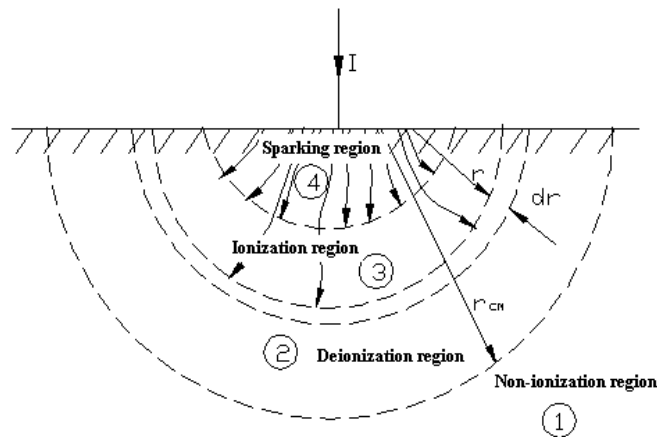
Σχήμα 1.5 Μοντέλο Wang – Liew – Darveniza.
