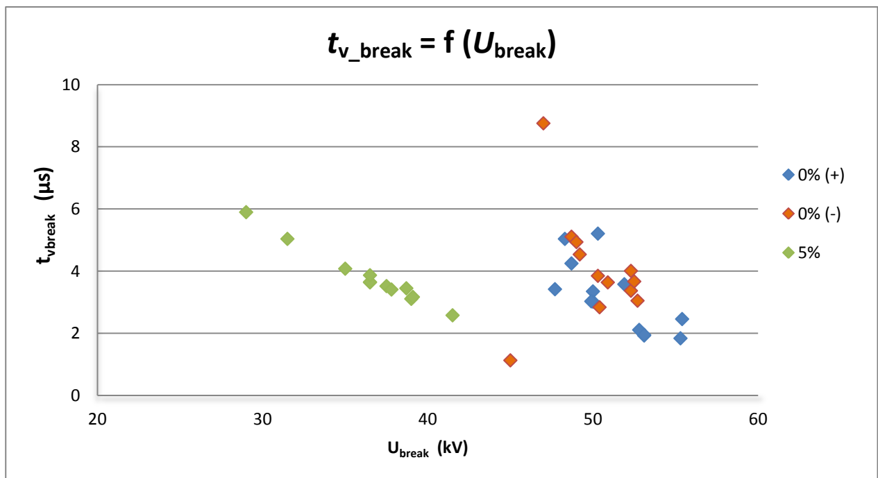
Γράφημα 4.18 Χρόνος διάσπασης συναρτήσει της τάσης διάσπασης για το δοκίμιο Δ'.
