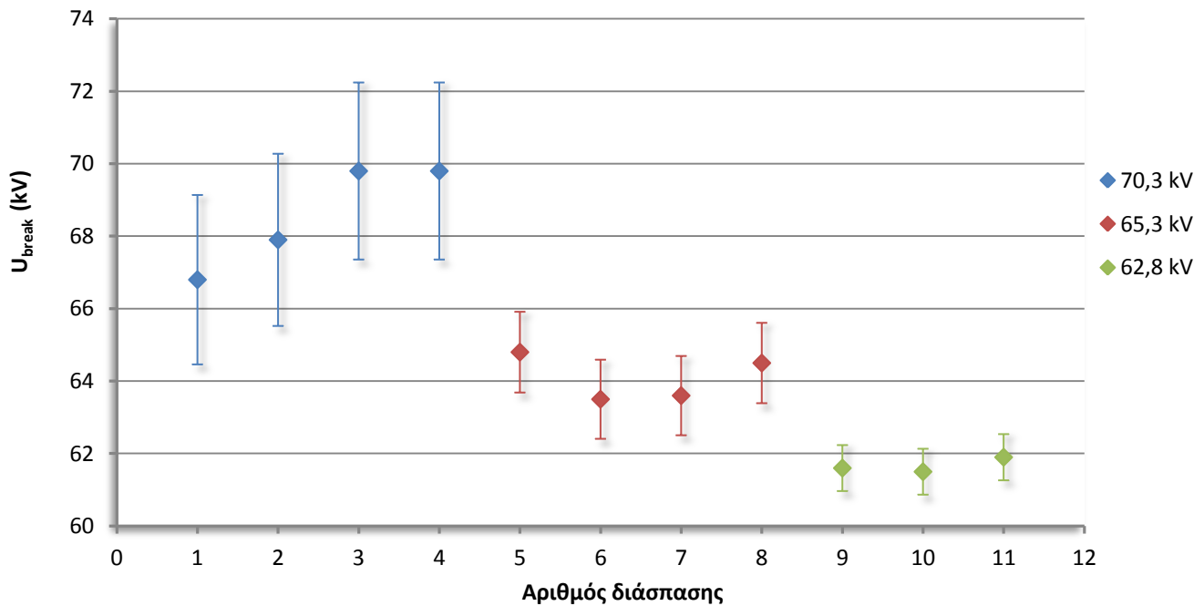
Γράφημα 4.2 Αβεβαιότητα τάσης τη στιγμή της διάσπασης ανά επίπεδο τάσης, για το δοκίμιο Β' 0% υγρασία, θετική πολικότητα.
