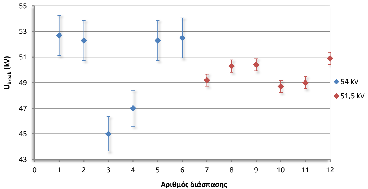
Γράφημα 4.12 Αβεβαιότητα τάσης τη στιγμή της διάσπασης ανά επίπεδο τάσης, για το δοκίμιο Δ' 0% υγρασία, αρνητική πολικότητα.
