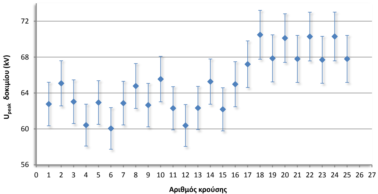
Γράφημα 4.1: Αβεβαιότητα τάσης δοκιμίου Β' 0% υγρασία, θετική πολικότητα.
