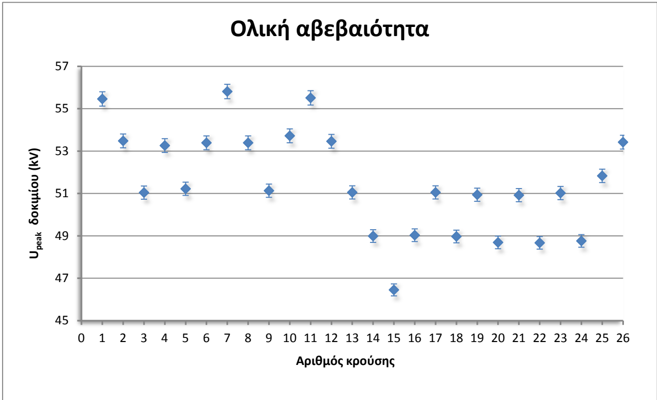
Γράφημα 4.9 Αβεβαιότητα τάσης δοκιμίου Δ' 0% υγρασία, θετική πολικότητα.
