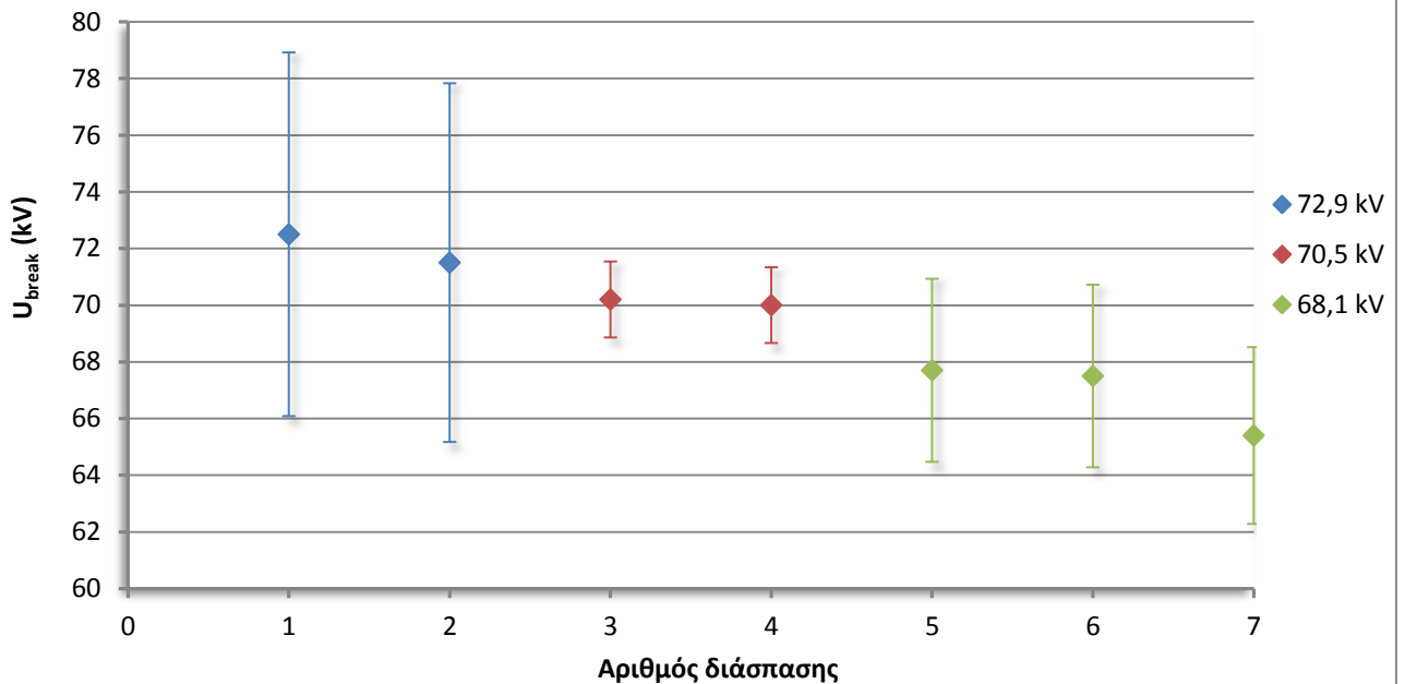
Γράφημα 4.4 Αβεβαιότητα τάσης τη στιγμή της διάσπασης ανά επίπεδο τάσης, για το δοκίμιο Β' 0% υγρασία, αρνητική πολικότητα.
