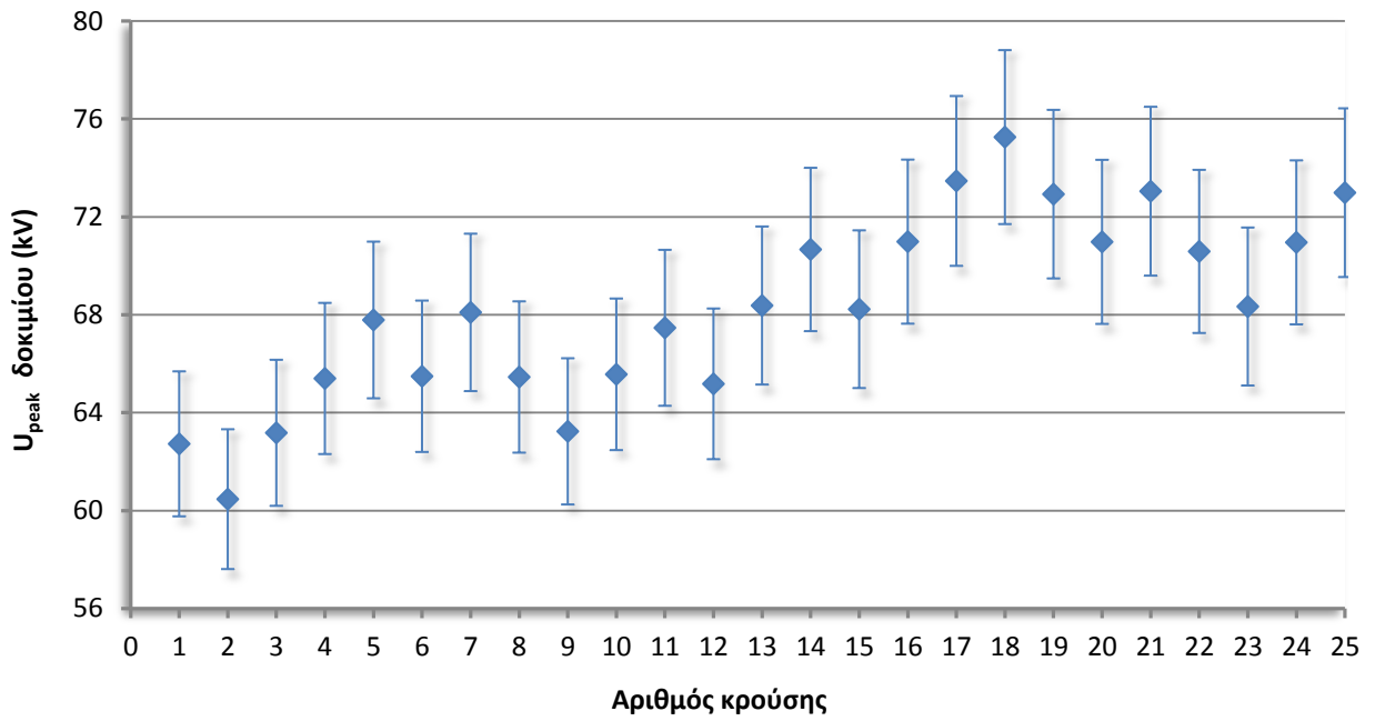
Γράφημα 4.3 Αβεβαιότητα τάσης δοκιμίου Β' 0% υγρασία, αρνητική πολικότητα.
