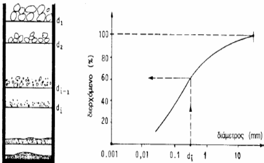
Σχήμα 2.10 Κοκκομέτρηση εδαφών με κόσκινα.
