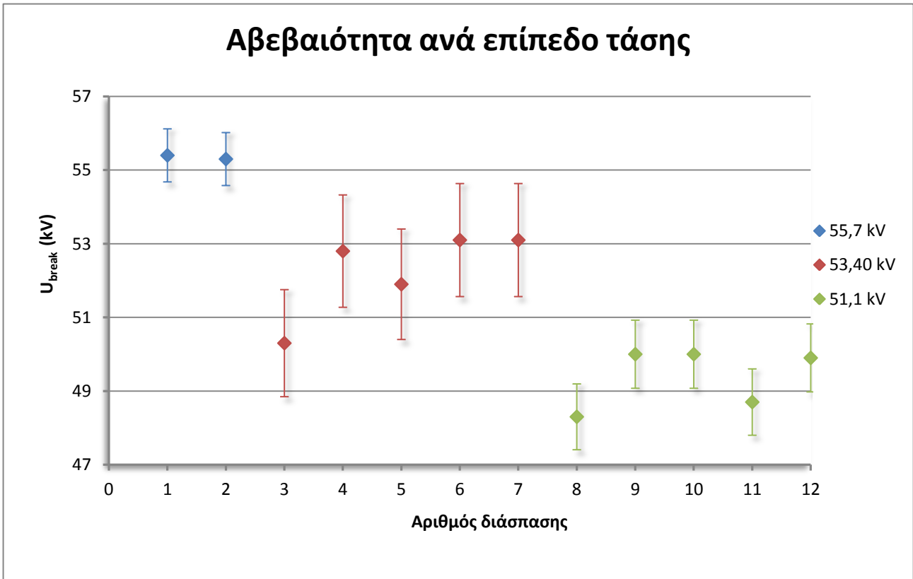
Γράφημα 4.10 Αβεβαιότητα τάσης τη στιγμή της διάσπασης ανά επίπεδο τάσης, για το δοκίμιο 0% υγρασία, θετική πολικότητα.
