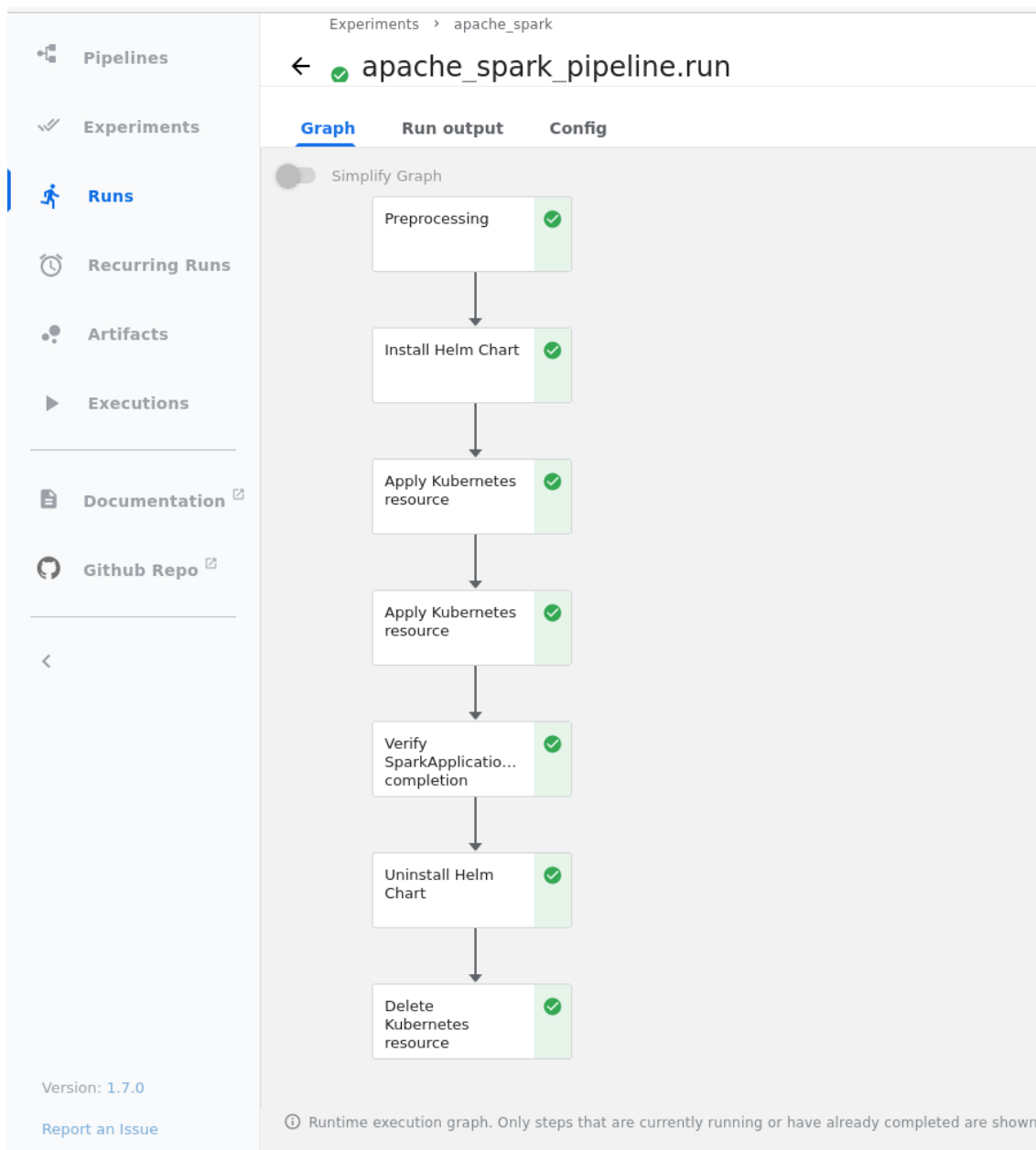
Σχήμα 4.1: Επιτυχημένη διοχέτευση KubeFlow
