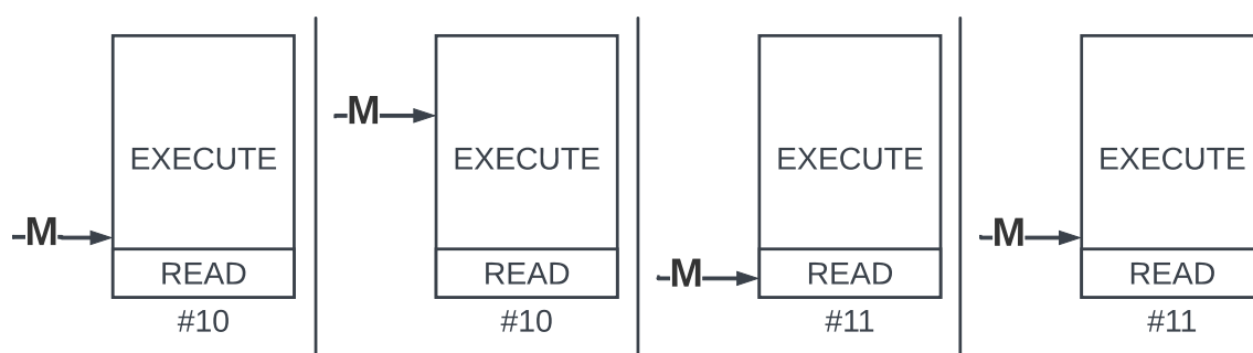
Σχήμα 5.10: Περίπτωση χωρίς προανάγνωση, το κύριο νήμα διαβάσει τα block.
