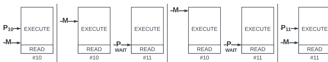
Σχήμα 5.11: Περίπτωση με RA=0 , το νήμα προανάγνωσης περιμένει το κύριο νήμα, αφού του διαβάσει το επόμενο block. Το state που βλέπουν οι predictors είναι επίκαιρο.
