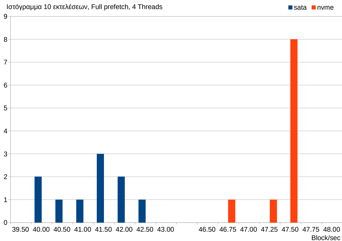
Σχήμα 6.5: Κατανομή της ταχύτητας εκτέλεσης των 10 ίδιων δοκιμών για κάθε δίσκο, με 4 βήματα προανάκτησης.
