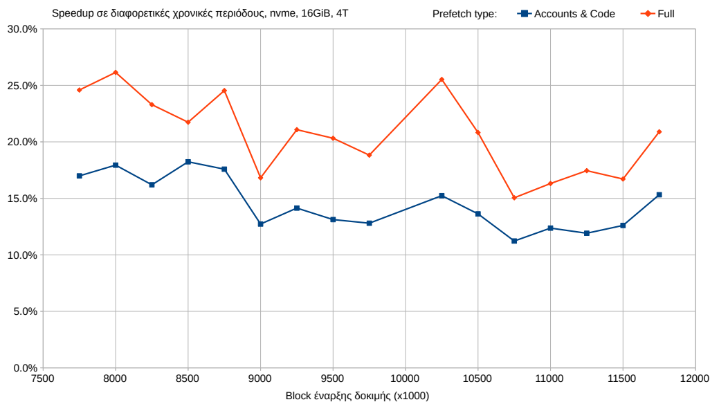
Σχήμα 7.9: Εξέλιξη του speedup ως προς την χρονική περίοδο δοκιμής. Ο άξονας ξεκινά από τον Απρίλιο του 2019 και τελειώνει με το Μάρτιο του 2021.
