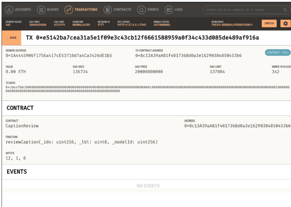
Εικόνα 13: Ganache - Ανάλυση καταχωρημένης συναλλαγής
