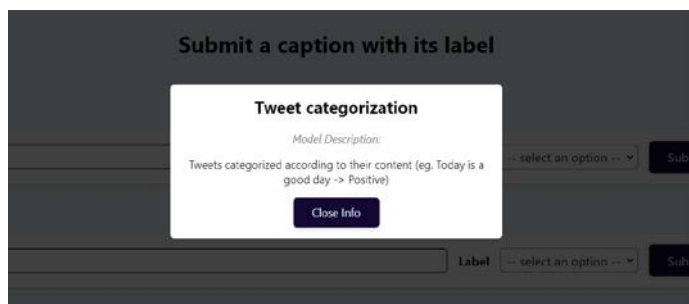
Εικόνα 25: DEMOS - Παράδειγμα ανάλυσης πληροφοριών μοντέλου NA
