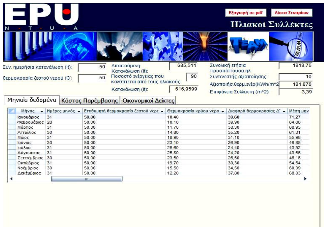
Εικόνα 4.30: Ηλιακοί συλλέκτες - Μηνιαία δεδομένα
