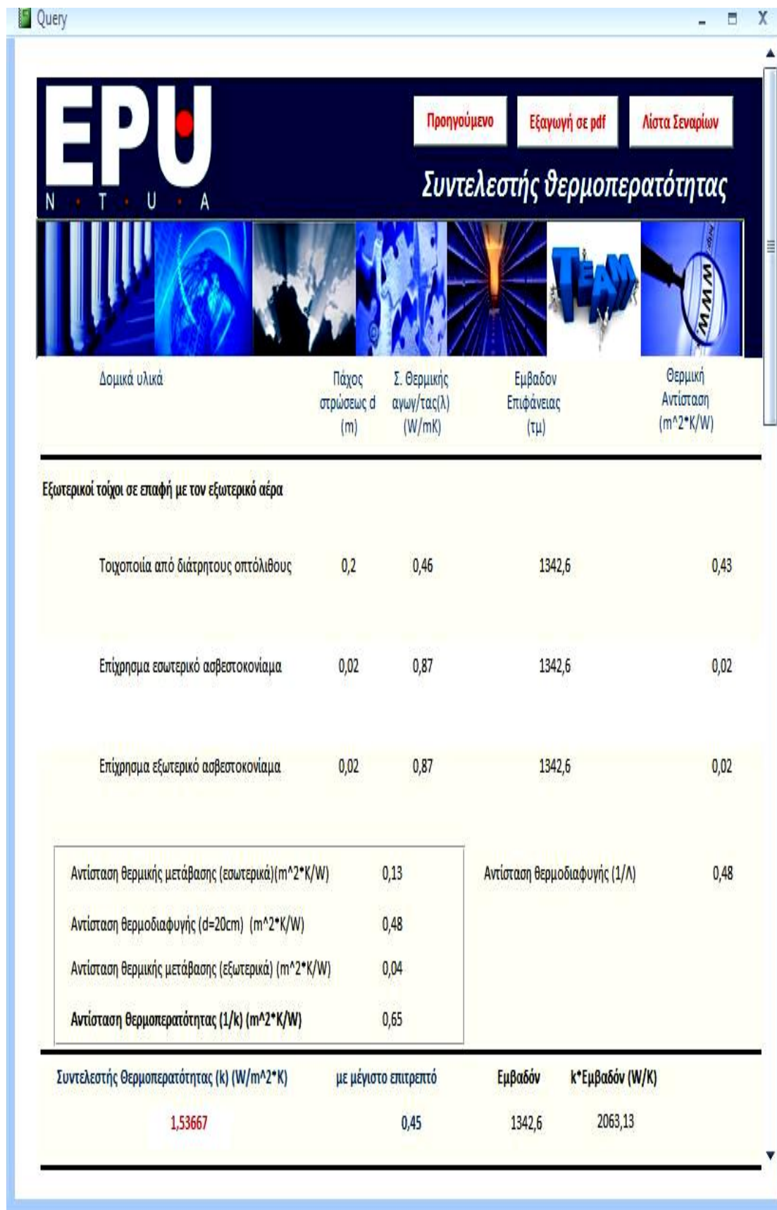
Εικόνα 4.15α: Υπολογισμός συντελεστή θερμοπερατότητας
