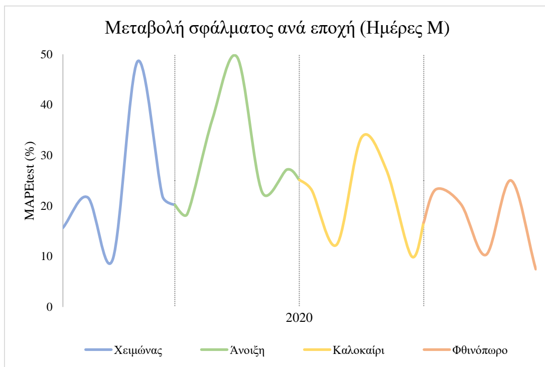
Σχήμα 5.11 : Σφάλματα προβλέψεων ημερών Μ για το μοντέλο ΜΔΥ Περδικούλα
