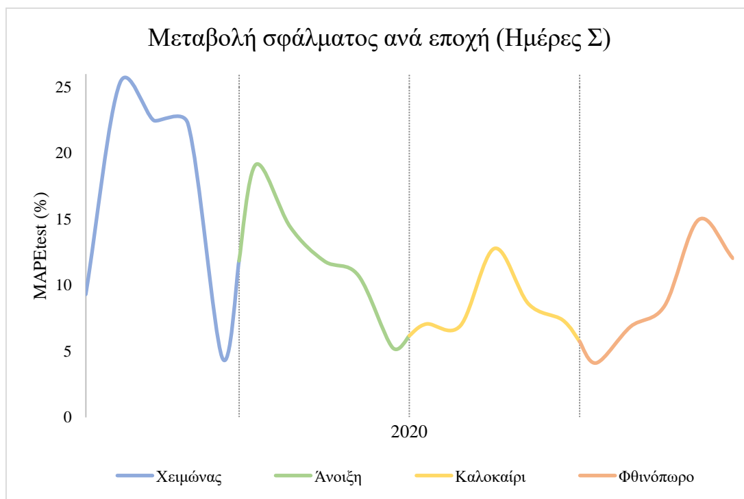
Σχήμα 5.10 : Σφάλματα προβλέψεων ημερών Σ για το μοντέλο ΜΔΥ Περδικούλα
