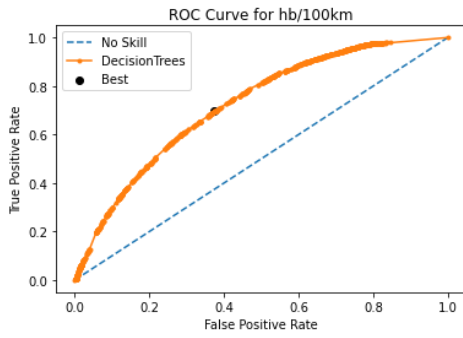
Γράφημα 5.22: Καμπύλη ROC αλγορίθμου Decision Trees για τις απότομες επιβραδύνσεις ανά 100χλμ.
