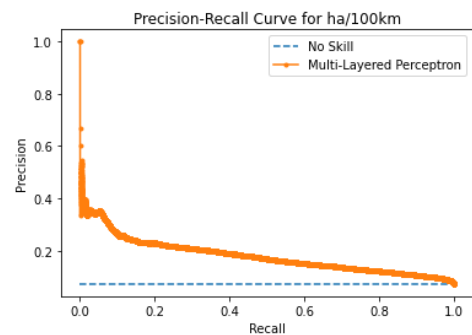
Γράφημα 5.62: Καμπύλη Ακρίβειας-Ανάκλησης αλγορίθμου MLP για τις απότομες επιταχύνσεις ανά 100χλμ.
