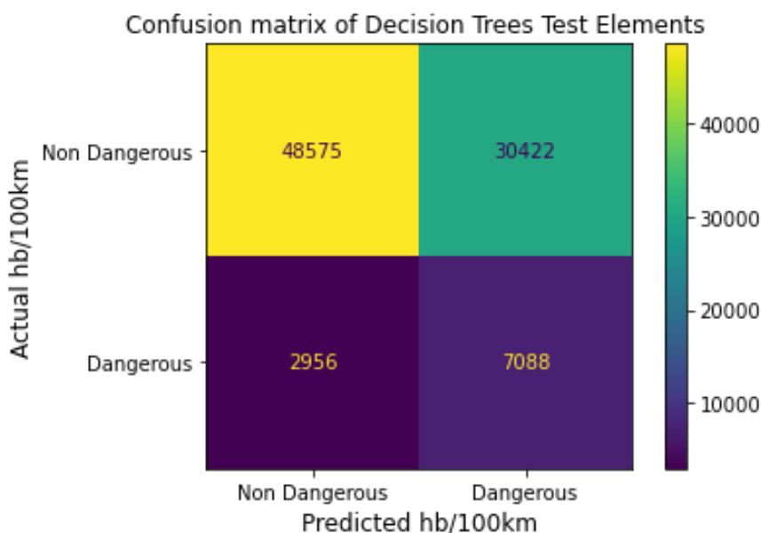
Γράφημα 5.21: Μήτρα σύγχυσης δεδομένων ελέγχου αλγορίθμου Decision Trees για τις απότομες επιβραδύνσεις ανά 100χλμ.
