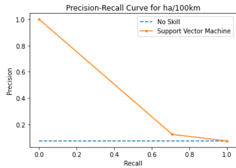
Γράφημα 5.56: Καμπύλη Ακρίβειας-Ανάκλησης αλγορίθμου SVM για τις απότομες επιταχύνσεις ανά 100χλμ.
