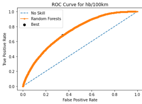
Γράφημα 5.40: Καμπύλη ROC αλγορίθμου Random Forests για τις απότομες επιβραδύνσεις ανά 100χλμ.
