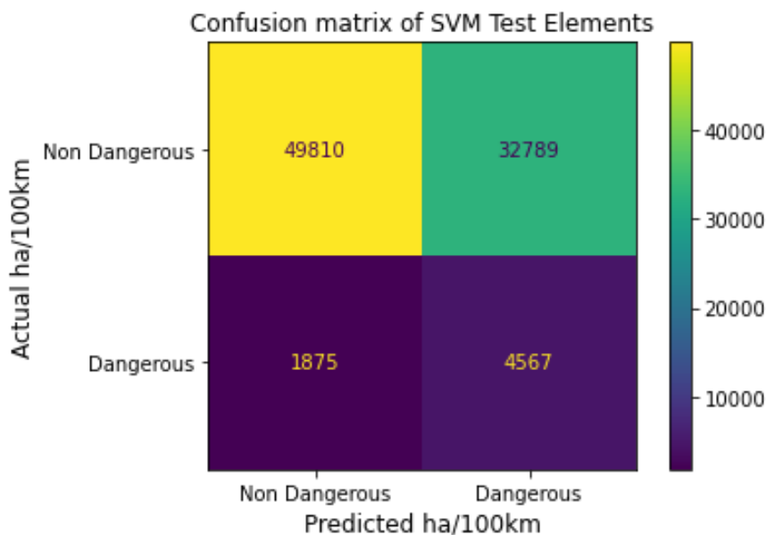
Γράφημα 5.54: Μήτρα σύγχυσης δεδομένων ελέγχου αλγόριθμου SVM για τις απότομες επιταχύνσεις ανά 100χλμ.
