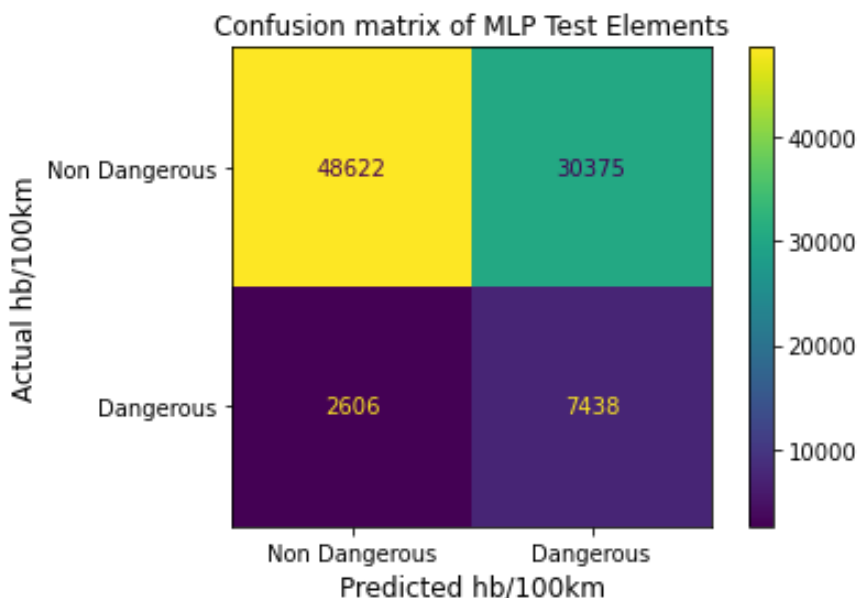
Γράφημα 5.63: Μήτρα σύγχυσης δεδομένων ελέγχου αλγορίθμου MLP για τις απότομες επιβραδύνσεις ανά 100χλμ.
