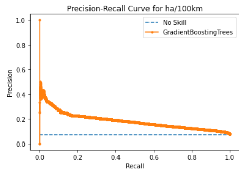
Γράφημα 5.26: Καμπύλη Ακρίβειας-Ανάκλησης αλγορίθμου Gradient Boosting για τις απότομες επιταχύνσεις ανά 100χλμ.
