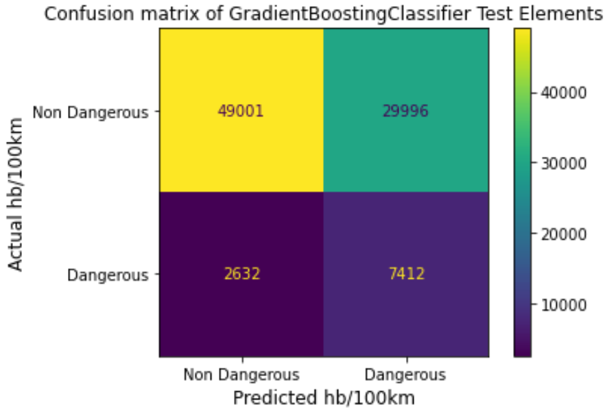
Γράφημα 5.27: Μήτρα σύγκρισης δεδομένων ελέγχου αλγορίθμου Gradient Boosting για τις απότομες επιβραδύνσεις ανά 100χλμ.
