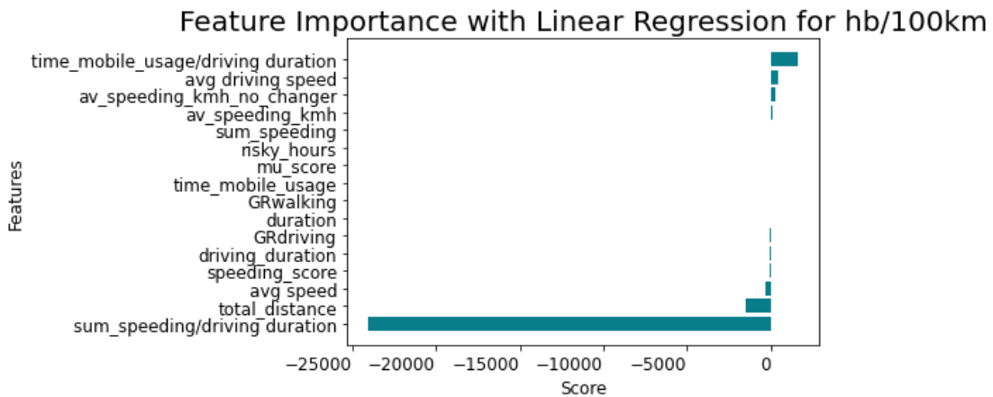
Γράφημα 5.2: Σημαντικότητα Χαρακτηριστικών για τις απότομες επιβραδύνσεις ανά 100χλμ. με Γραμμική Παλινδρόμηση
