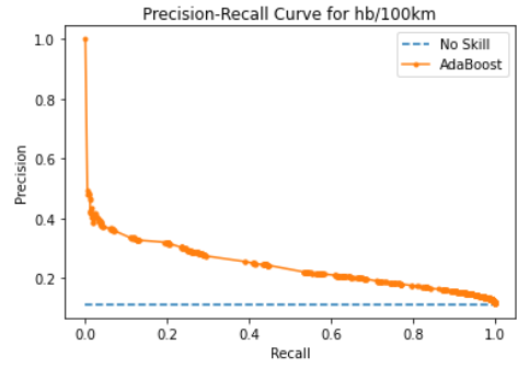
Γράφημα 5.47: Καμπύλη Ακρίβειας-Ανάκλησης αλγορίθμου AdaBoost για τις απότομες επιβραδύνσεις ανά 100χλμ.
