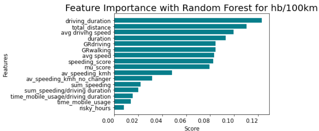
Γράφημα 5.6: Σημαντικότητα Χαρακτηριστικών για τις απότομες επιβραδύνσεις ανά 100χλμ. με Random Forests
