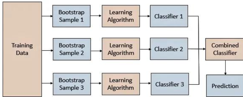
Εικόνα 3.6: Διάγραμμα Ροής αλγορίθμου Bootstrap Aggregation
