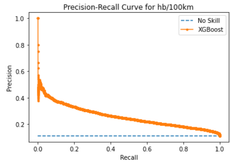
Γράφημα 5.35: Καμπύλη Ακρίβειας-Ανάκλησης αλγορίθμου XGBoost για τις απότομες επιβραδύνσεις ανά 100χλμ.
