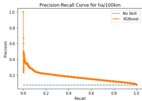
Γράφημα 5.32: Καμπύλη Ακρίβειας-Ανάκλησης αλγορίθμου XGBoost για τις απότομες επιταχύνσεις ανά 100χλμ.
