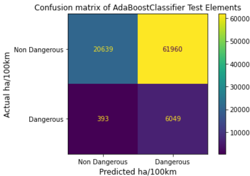
Γράφημα 5.42: Μήτρα σύγκρισης δεδομένων ελέγχου αλγορίθμου AdaBoost για τις απότομες επιταχύνσεις ανά 100χλμ.
