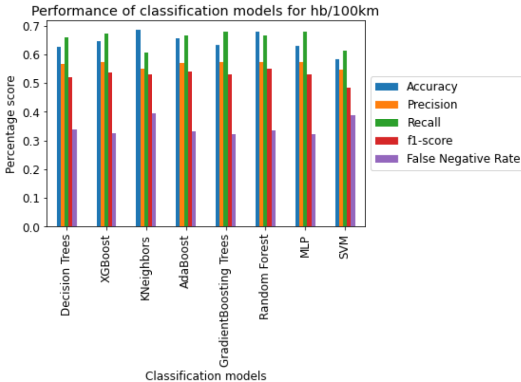
Γράφημα 6.2: Σύγκριση μετρικών αποτελεσμάτων των μοντέλων ταξινόμησης για τις απότομες επιβραδύνσεις ανά 100χλμ.
