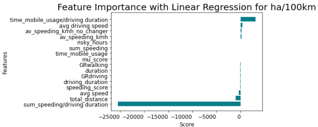
Γράφημα 5.1: Σημαντικότητα Χαρακτηριστικών για τις απότομες επιταχύνσεις ανά 100χλμ. με Γραμμική Παλινδρόμηση
