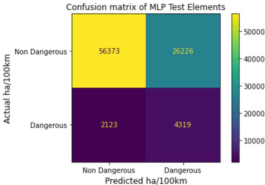
Γράφημα 5.60: Μήτρα σύγκρισης δεδομένων ελέγχου αλγορίθμου MLP για τις απότομες επιταχύνσεις ανά 100χλμ.
