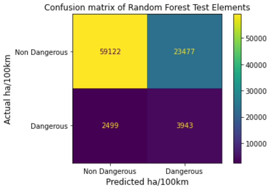
Γράφημα 5.36: Μήτρα σύγχυσης δεδομένων ελέγχου αλγορίθμου Random Forests για τις απότομες επιταχύνσεις ανά 100χλμ.
