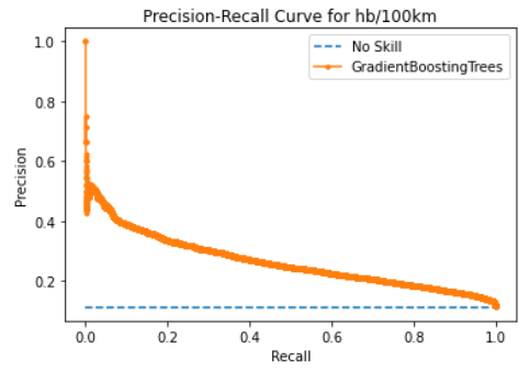
Γράφημα 5.29: Καμπύλη Ακρίβειας-Ανάκλησης αλγορίθμου Gradient Boosting για τις απότομες επιβραδύνσεις ανά 100χλμ.
