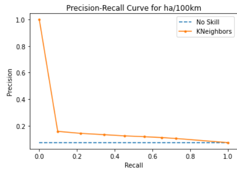
Γράφημα 5.50: Καμπύλη Ακρίβειας-Ανάκλησης αλγόριθμου KNN για τις απότομες επιταχύνσεις ανά 100χλμ.
