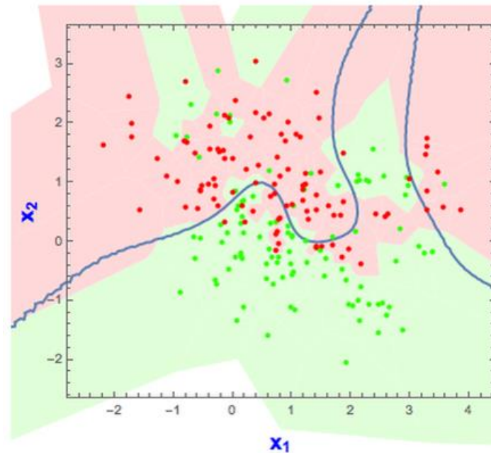
Εικόνα 3.10: Οπτικοποίηση αλγορίθμου K-πλησιέστερων γειτόνων με διάγραμμα Voronoi
