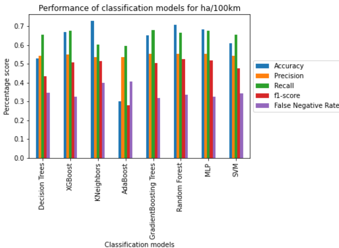
Γράφημα 6.1: Σύγκριση μετρικών αποτελεσμάτων των μοντέλων ταξινόμησης για τις απότομες επιταχύνσεις ανά 100χλμ.
