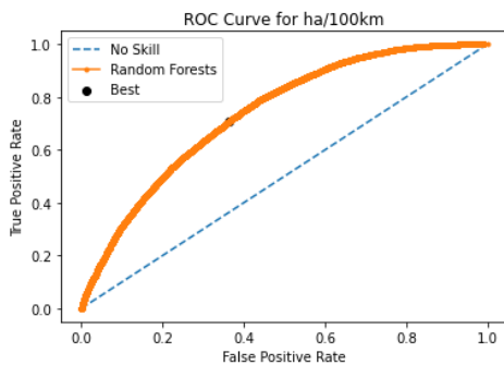
Γράφημα 5.37: Καμπύλη ROC αλγορίθμου Random Forests για τις απότομες επιταχύνσεις ανά 100χλμ.
