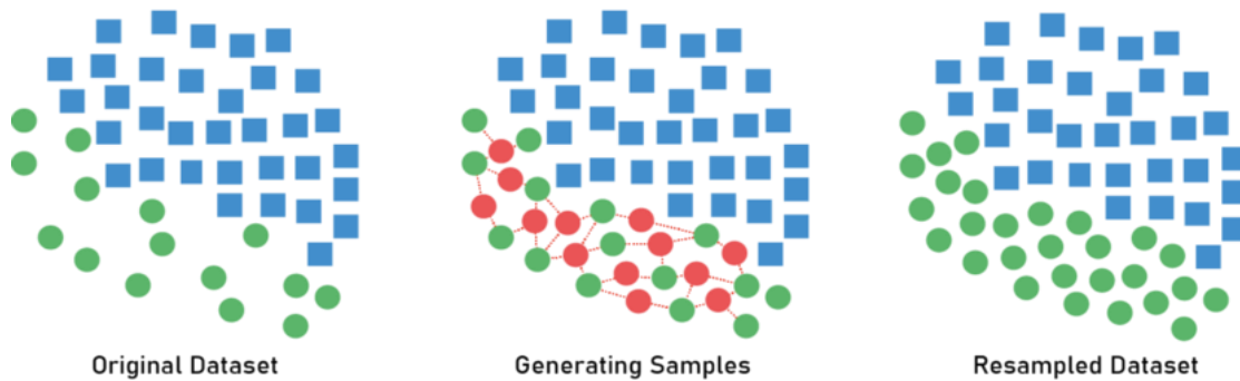
Εικόνα 3.19: Τεχνηκή Συνθετική Μειονοτικής Υπερδειγματοληψίας (SMOTE)
