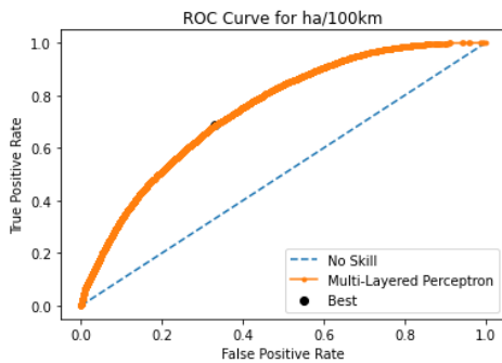
Γράφημα 5.61: Καμπύλη ROC αλγορίθμου MLP για τις απότομες επιταχύνσεις ανά 100χλμ.
