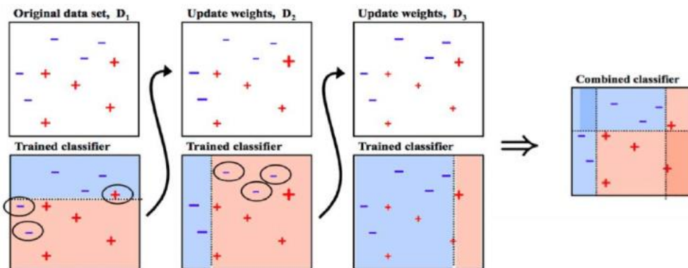
Εικόνα 3.7: Διάγραμμα Ροής εκπαίδευσης αλγορίθμου AdaBoost
