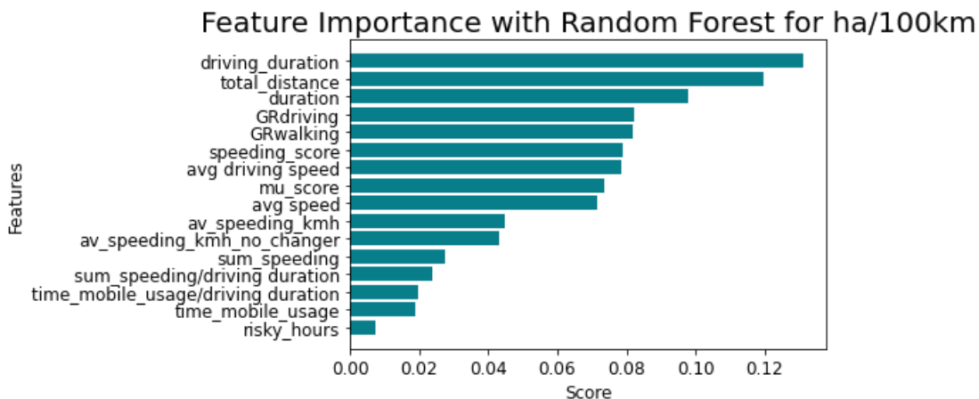
Γράφημα 5.5: Σημαντικότητα Χαρακτηριστικών για τις απότομες επιταχύνσεις ανά 100χλμ. με Random Forests
