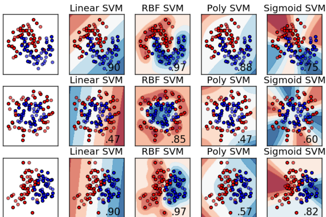
Εικόνα 3.12: Ταξινόμηση με SVM εφαρμόζοντας εναλλακτικές Μεθόδους Πυρήνα
