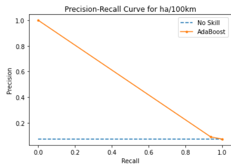
Γράφημα 5.44: Καμπύλη Ακρίβειας-Ανάκλησης αλγορίθμου AdaBoost για τις απότομες επιταχύνσεις ανά 100χλμ.
