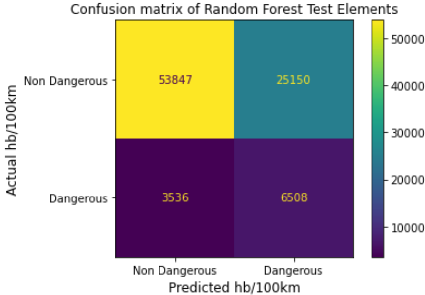
Γράφημα 5.39: Μήτρα σύγχυσης δεδομένων ελέγχου αλγορίθμου Random Forests για τις απότομες επιβραδύνσεις ανά 100χλμ.
