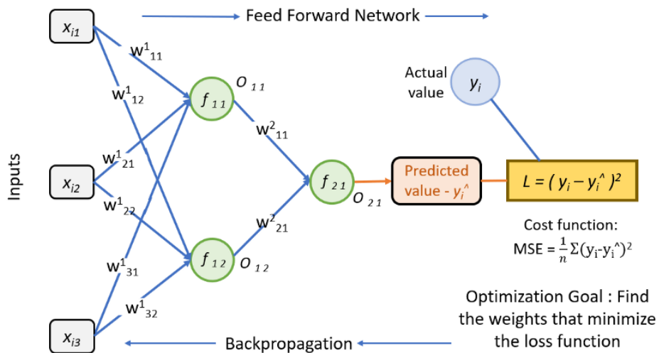
Εικόνα 3.15: Διάγραμμα ροής Πολυεπίπεδου Αισθητήρα NN (MLP NN)
