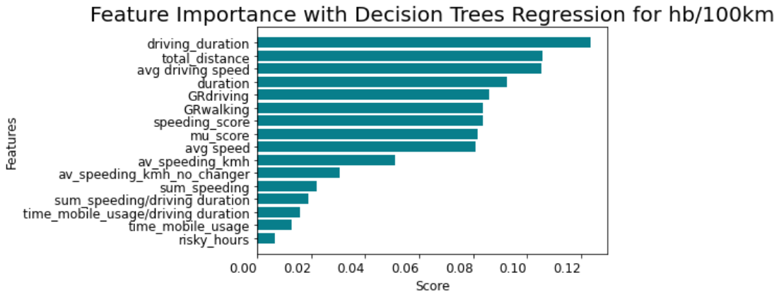
Γράφημα 5.4: Σημαντικότητα Χαρακτηριστικών για τις απότομες επιβραδύνσεις ανά 100χλμ. με Decision Trees
