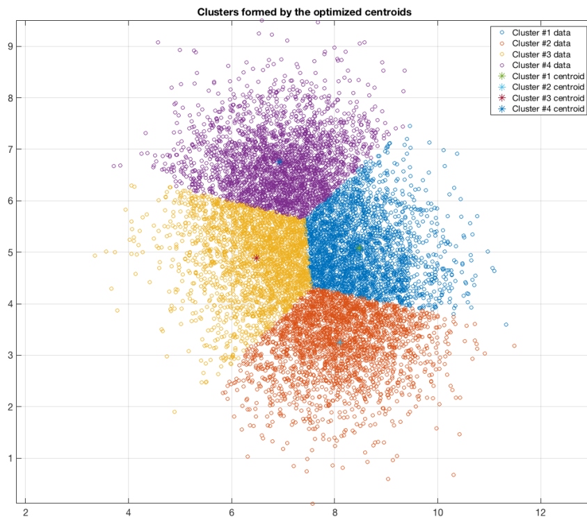
Εικόνα 3.17: Τοπική οπτικοποίηση ομαδοποίησης με αλγόριθμο K-μέσου 4 κεντροειδών
