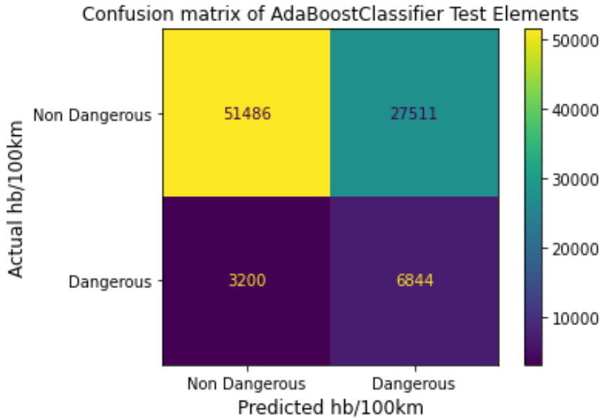
Γράφημα 5.45: Μήτρα σύγχυσης δεδομένων ελέγχου αλγορίθμου AdaBoost για τις απότομες επιβραδύνσεις ανά 100χλμ.
