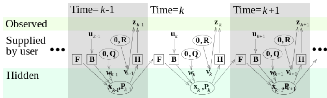
Εικόνα 4.2: Συγχώνευση δεδομένων με φίλτρο Kalman πολλαπλών διαστάσεων
