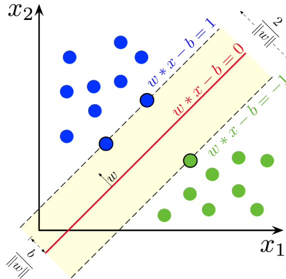
Εικόνα 3.11: Απεικόνιση βέλτιστου υπερεπιπέδου δεδομένων δύο κλάσεων σε διδιάστατο χώρο
