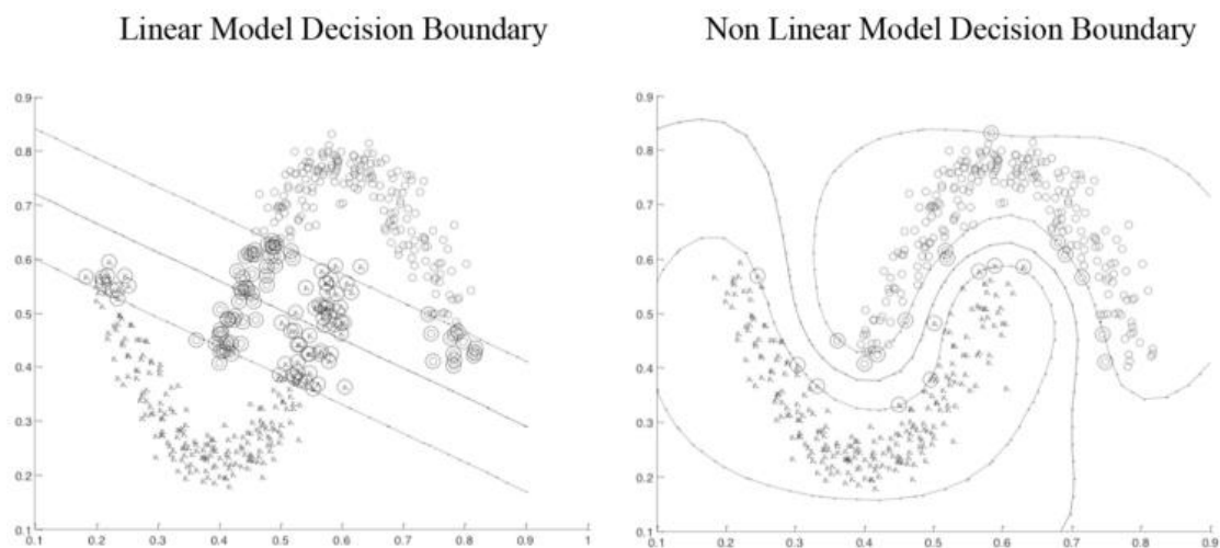
Εικόνα 3.13: Διαχωρισμός πυρήνα μεταξύ Γραμμικού και Μη γραμμικού πολυδιάστατου μοντέλου SVM
