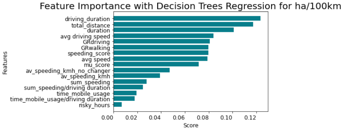
Γράφημα 5.3: Σημαντικότητα Χαρακτηριστικών για τις απότομες επιταχύνσεις ανά 100χλμ. με Decision Trees
