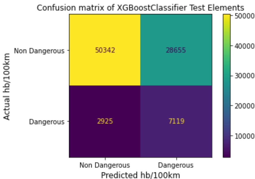
Γράφημα 5.33: Μήτρα σύγχυσης δεδομένων ελέγχου αλγορίθμου XGBoost για τις απότομες επιβραδύνσεις ανά 100χλμ.
