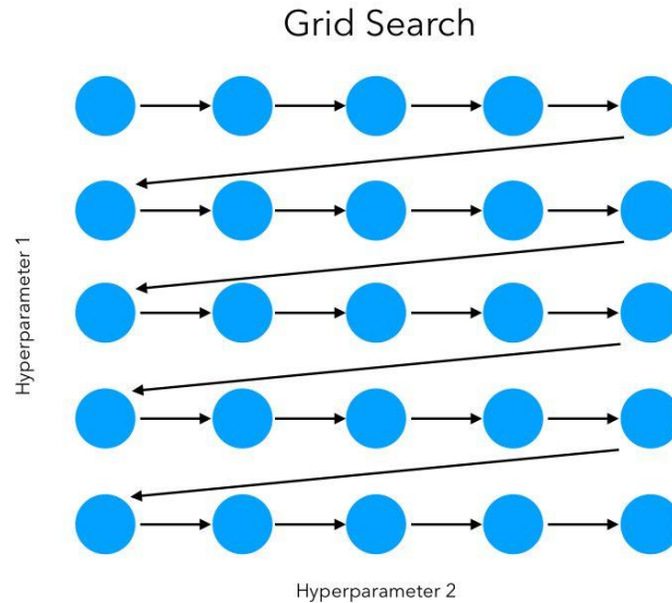
Εικόνα 3.20: Αλληλουχία διαδικασίας συντονισμού δύο υπερπαραμέτρων με την αναζήτηση πλέγματος
