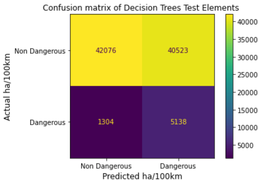
Γράφημα 5.18: Μήτρα σύγχυσης δεδομένων ελέγχου αλγορίθμου Decision Trees για τις απότομες επιταχύνσεις ανά 100χλμ.
