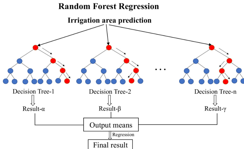
Εικόνα 3.5: Τυπικό διάγραμμα αλγορίθμου Random Forests
