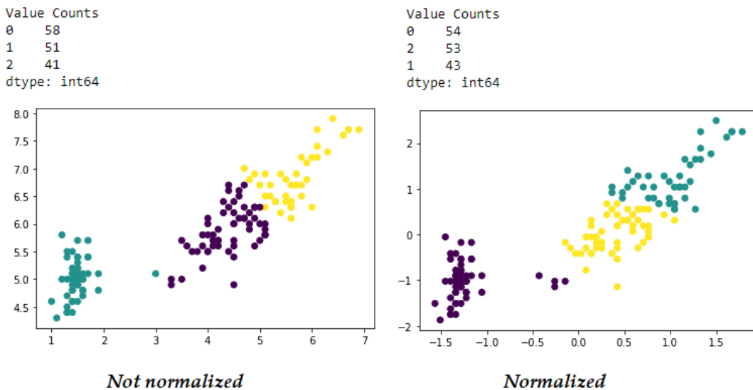
Εικόνα 3.16: Διαφορές ομαδοποίησης δεδομένων πριν και μετά την κανονικοποίηση
