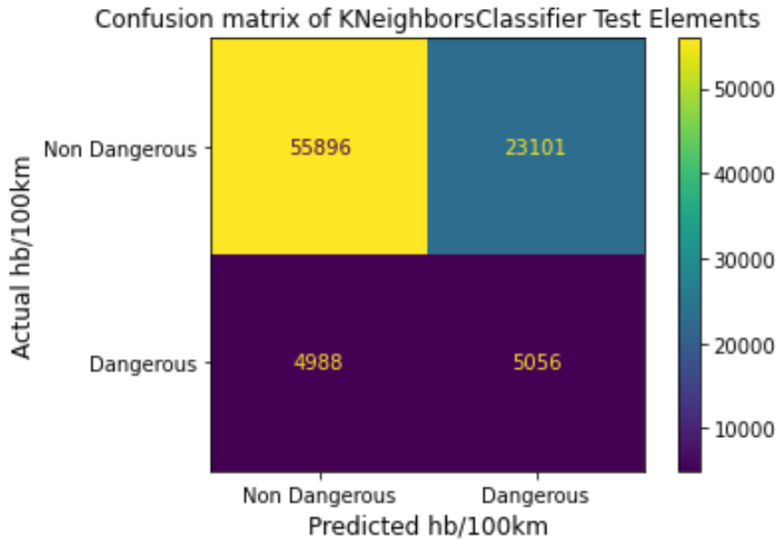
Γράφημα 5.51: Μήτρα σύγχυσης δεδομένων ελέγχου αλγορίθμου KNN για τις απότομες επιβραδύνσεις ανά 100χλμ.
