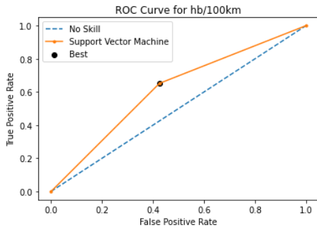
Γράφημα 5.58: Καμπύλη ROC αλγορίθμου SVM για τις απότομες επιβραδύνσεις ανά 100χλμ.
