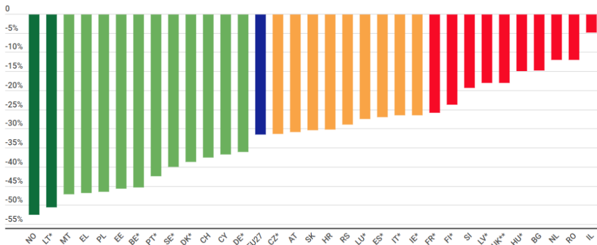
Γράφημα 1.2: Σχετικές μεταβολές (%) στα θανατηφόρα ατυχήματα στην Ευρώπη (2011-2021)
