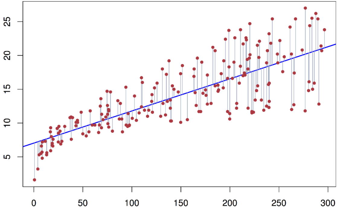
Εικόνα 3.1: Μοντελοποίηση Γραμμικής Παλινδρόμησης σε δισδιάστατο χώρο
