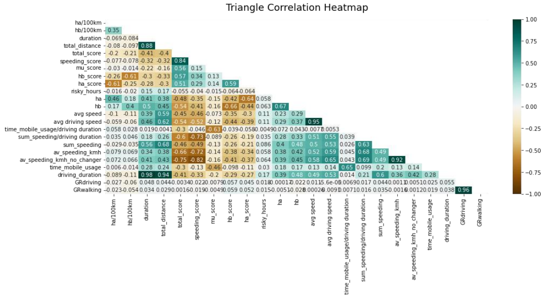
Γράφημα Περίληψης 1: Συντελεστής συσχέτισης Pearson των εξετασθέντων δεδομένων
