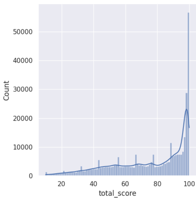
Γράφημα 4.4: Διακύμανση του συνολικού σκορ διαδρομής
