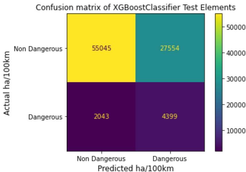
Γράφημα 5.30: Μήτρα σύγκρισης δεδομένων ελέγχου αλγορίθμου XGBoost για τις απότομες επιταχύνσεις ανά 100χλμ.
