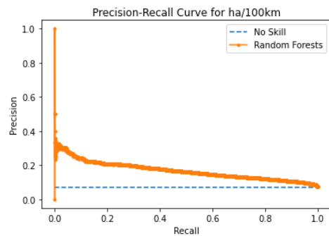
Γράφημα 5.38: Καμπύλη Ακρίβειας-Ανάκλησης αλγορίθμου Random Forests για τις απότομες επιταχύνσεις ανά 100χλμ.
