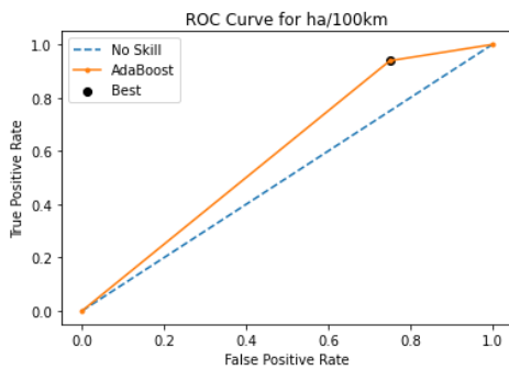
Γράφημα 5.43: Καμπύλη ROC αλγορίθμου AdaBoost για τις απότομες επιταχύνσεις ανά 100χλμ.
