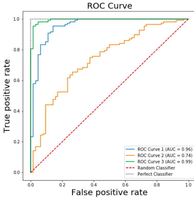
Εικόνα 3.22: Καμπύλες ROC και τιμές AUC σε ταξινόμηση πολλαπλών κλάσεων
