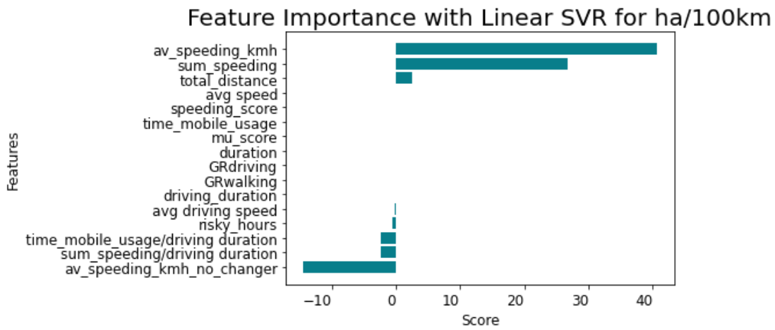
Γράφημα 5.9: Σημαντικότητα Χαρακτηριστικών για τις απότομες επιταχύνσεις ανά 100χλμ. με Linear SVR
