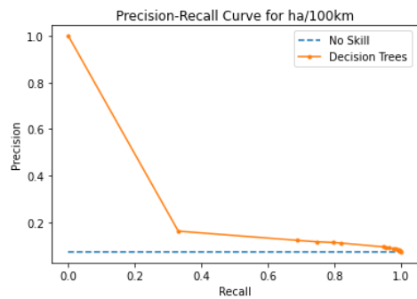
Γράφημα 5.20: Καμπύλη Ακρίβειας-Ανάκλησης αλγόριθμου Decision Trees για τις απότομες επιταχύνσεις ανά 100χλμ.
