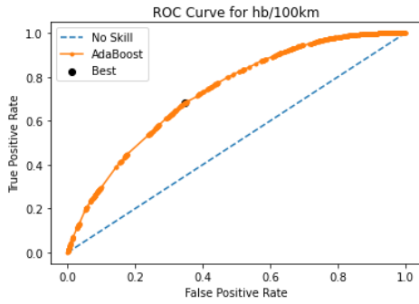
Γράφημα 5.46: Καμπύλη ROC αλγορίθμου AdaBoost για τις απότομες επιβραδύνσεις ανά 100χλμ.
