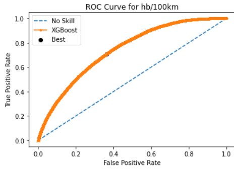
Γράφημα 5.34: Καμπύλη ROC αλγορίθμου XGBoost για τις απότομες επιβραδύνσεις ανά 100χλμ.
