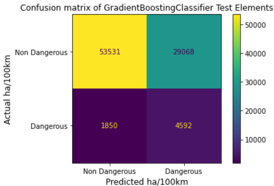
Γράφημα 5.24: Μήτρα σύγκρισης δεδομένων ελέγχου αλγορίθμου Gradient Boosting για τις απότομες επιταχύνσεις ανά 100χλμ.
