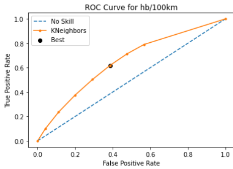
Γράφημα 5.52: Καμπύλη ROC αλγόριθμου KNN για τις απότομες επιβραδύνσεις ανά 100χλμ.
