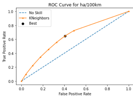
Γράφημα 5.49: Καμπύλη ROC αλγόριθμου KNN για τις απότομες επιταχύνσεις ανά 100χλμ.
