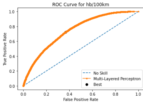
Γράφημα 5.64: Καμπύλη ROC αλγορίθμου MLP για τις απότομες επιβραδύνσεις ανά 100χλμ.
