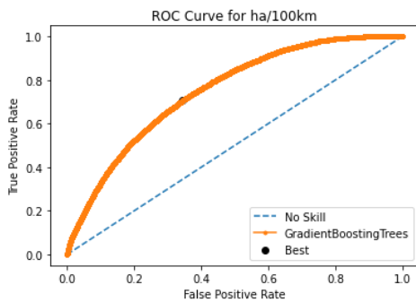
Γράφημα 5.25: Καμπύλη ROC αλγορίθμου Gradient Boosting για τις απότομες επιταχύνσεις ανά 100χλμ.
