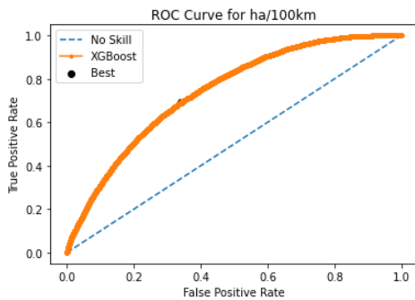
Γράφημα 5.31: Καμπύλη ROC αλγορίθμου XGBoost για τις απότομες επιταχύνσεις ανά 100χλμ.
