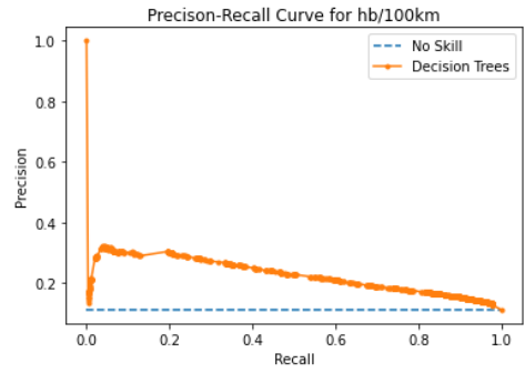
Γράφημα 5.23: Καμπύλη Ακρίβειας-Ανάκλησης αλγορίθμου Decision Trees για τις απότομες επιβραδύνσεις ανά 100χλμ.
