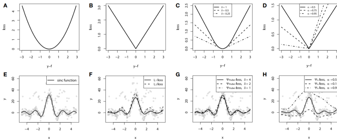
Εικόνα 3.8: Συνήθειες Συνεχείς Συναρτήσεις Απωλειών στην Ενίσχυση Κλίσης: (A) L_2 squared; (B) L_1 absolute; (C) Huber loss function; (D) Quantile loss function,
