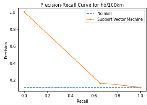
Γράφημα 5.59: Καμπύλη Ακρίβειας-Ανάκλησης αλγορίθμου SVM για τις απότομες επιβραδύνσεις ανά 100χλμ.
