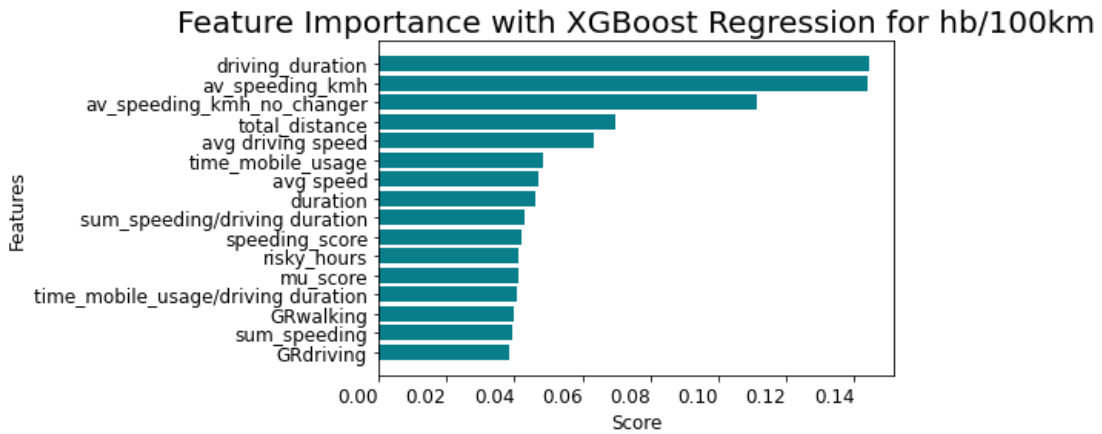
Γράφημα 5.8: Σημαντικότητα Χαρακτηριστικών για τις απότομες επιβραδύνσεις ανά 100χλμ. με XGBoost
