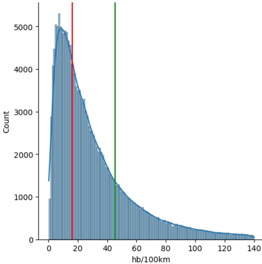
Γράφημα 5.12: Κεντροειδή και εύρεση threshold για τις απότομες επιβραδύνσεις ανά 100χλμ. με αλγόριθμο K-μέσου
