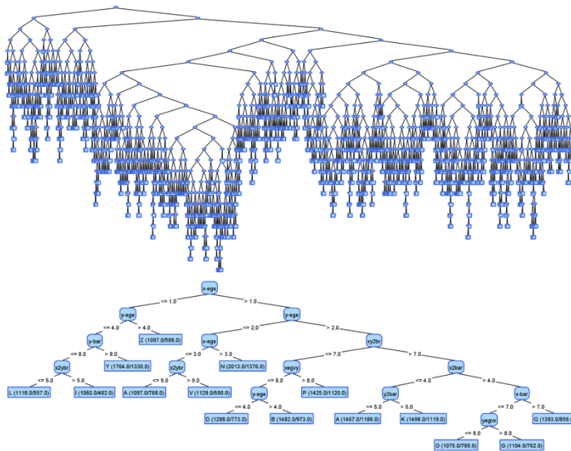
Εικόνα 3.4: Τυπικό διάγραμμα Decision Trees
