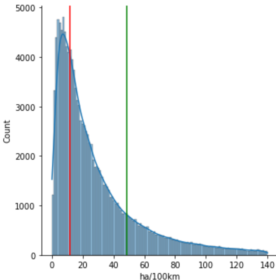
Γράφημα 5.11: Κεντροειδή και εύρεση threshold για τις απότομες επιταχύνσεις ανά 100χλμ. με αλγόριθμο K-μέσου
