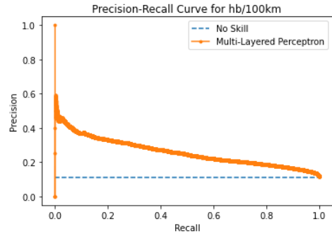
Γράφημα 5.65: Καμπύλη Ακρίβειας-Ανάκλησης αλγορίθμου MLP για τις απότομες επιβραδύνσεις ανά 100χλμ.
