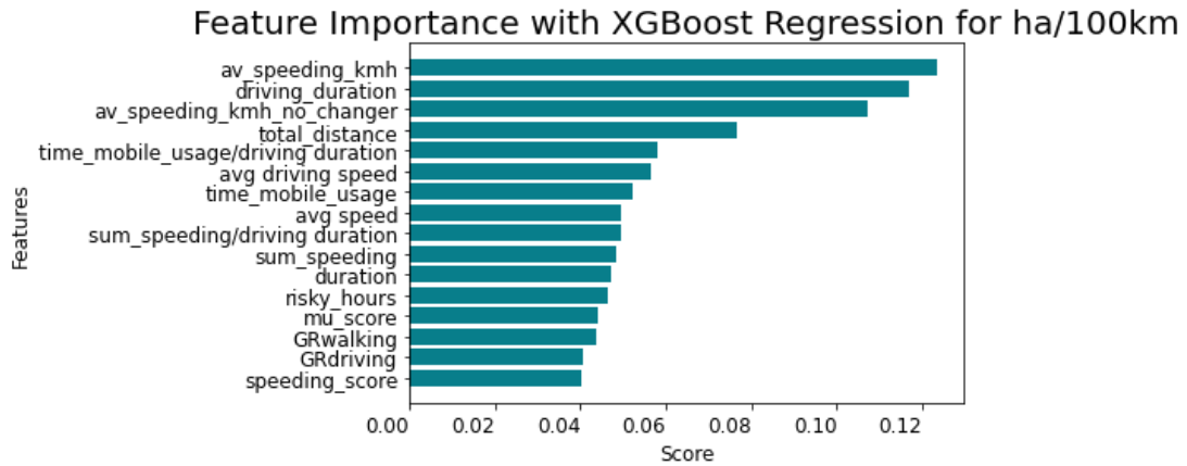
Γράφημα 5.7: Σημαντικότητα Χαρακτηριστικών για τις απότομες επιταχύνσεις ανά 100χλμ. με XGBoost
