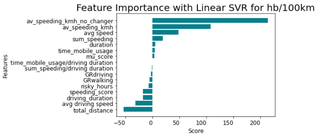
Γράφημα 5.10: Σημαντικότητα Χαρακτηριστικών για τις απότομες επιβραδύνσεις ανά 100χλμ. με Linear SVR
