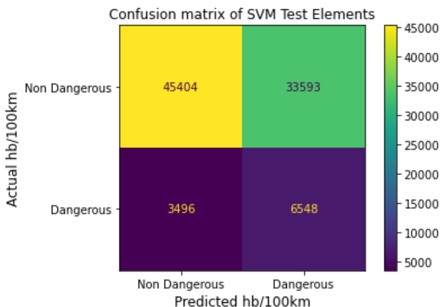
Γράφημα 5.57: Μήτρα σύγχυσης δεδομένων ελέγχου αλγορίθμου SVM για τις απότομες επιβραδύνσεις ανά 100χλμ.
