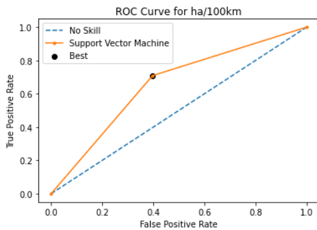
Γράφημα 5.55: Καμπύλη ROC αλγορίθμου SVM για τις απότομες επιταχύνσεις ανά 100χλμ.
