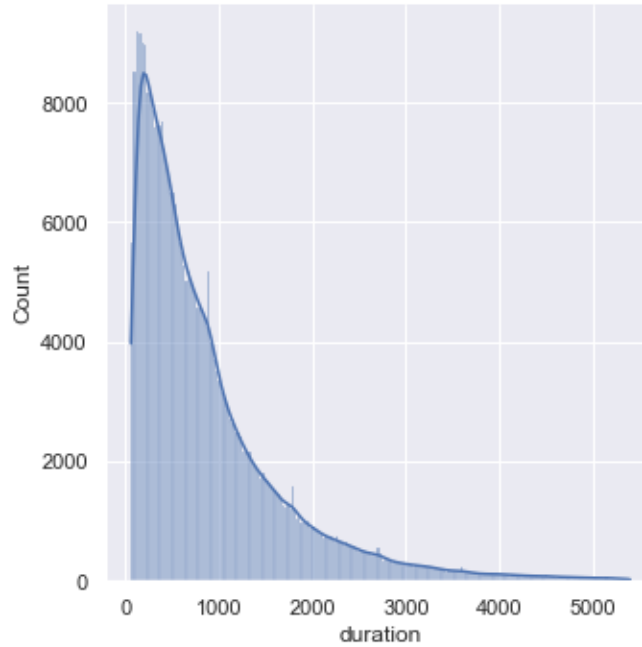
Γράφημα 4.1: Διακύμανση της κατανομής της διάρκειας διαδρομής
