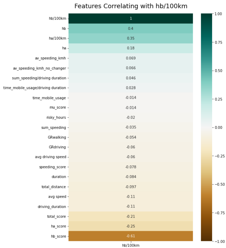
Γράφημα 4.7: Συσχέτιση Pearson ανεξάρτητων μεταβλητών με απότομες επιβραδύνσεις ανά 100 χλμ.
