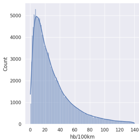
Γράφημα 4.3: Διακύμανση απότομων επιβραδύνσεων ανά 100χλμ.
