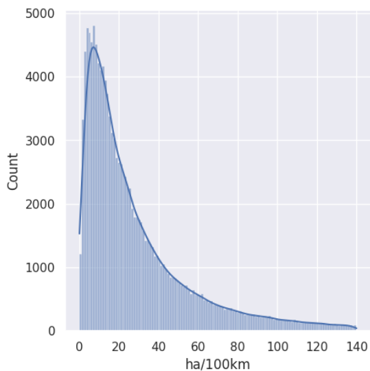
Γράφημα 4.2: Διακύμανση απότομων επιταχύνσεων ανά 100χλμ.
