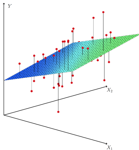
Εικόνα 3.2: Μοντελοποίηση πολυμεταβλητής Γραμμικής Παλινδρόμησης σε τρισδιάστατο χώρο
