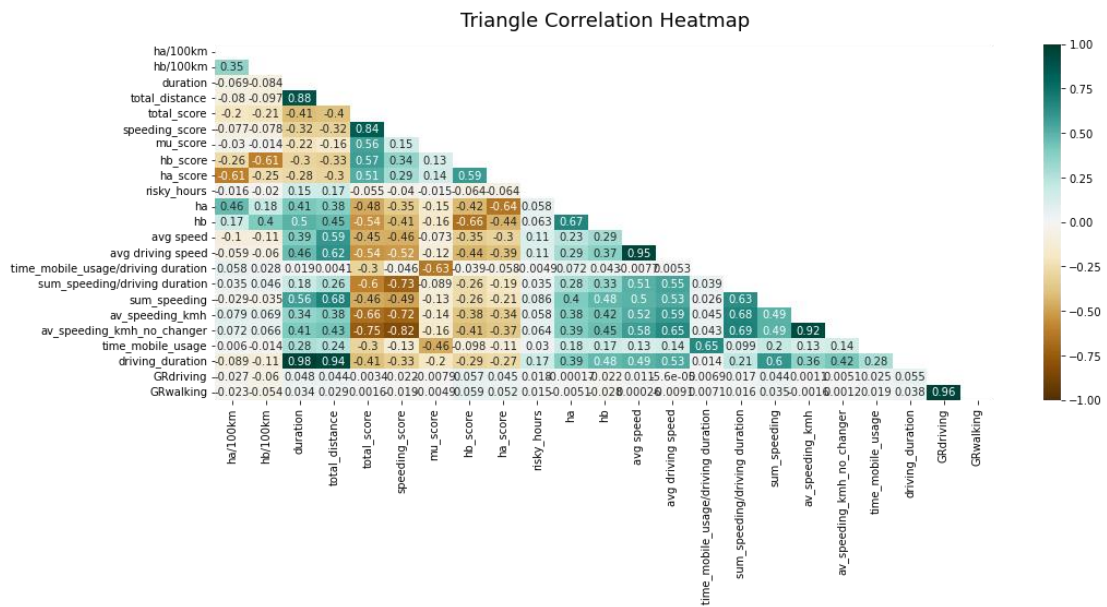
Γράφημα 4.5: Τριγωνικός πίνακας θερμότητας συσχέτισης μεταβλητών κατά Pearson
