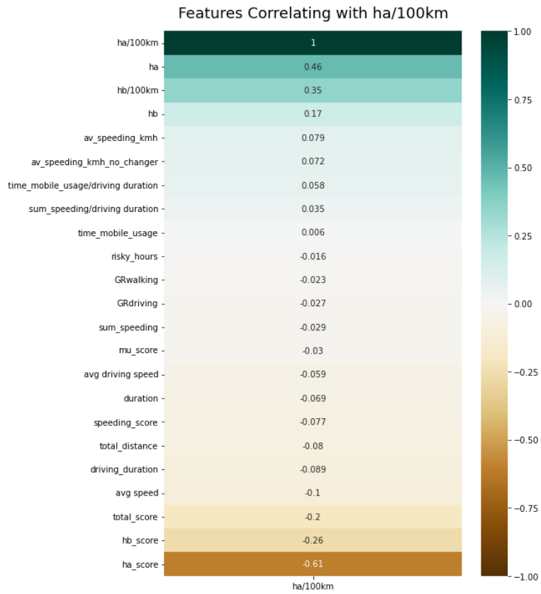
Γράφημα 4.6: Συσχέτιση Pearson ανεξάρτητων μεταβλητών με απότομες επιταχύνσεις ανά 100 χλμ.
