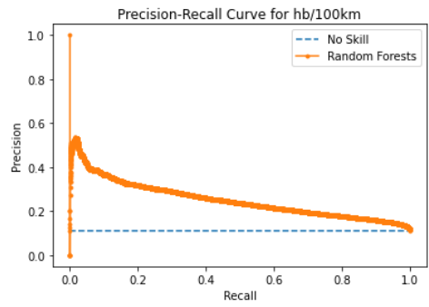
Γράφημα 5.41: Καμπύλη Ακρίβειας-Ανάκλησης αλγορίθμου Random Forests για τις απότομες επιβραδύνσεις ανά 100χλμ.
