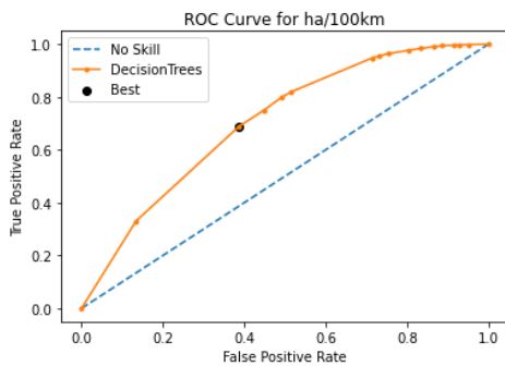
Γράφημα 5.19: Καμπύλη ROC αλγόριθμου Decision Trees για τις απότομες επιταχύνσεις ανά 100χλμ.
