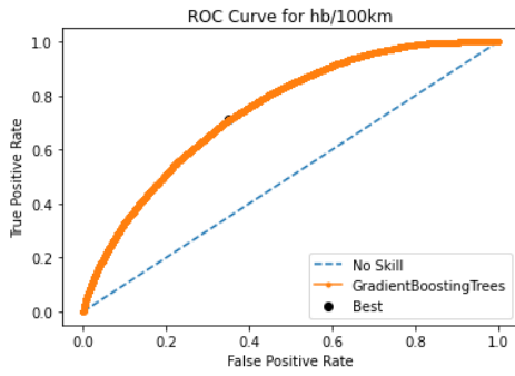
Γράφημα 5.28: Καμπύλη ROC αλγορίθμου Gradient Boosting για τις απότομες επιβραδύνσεις ανά 100χλμ.
