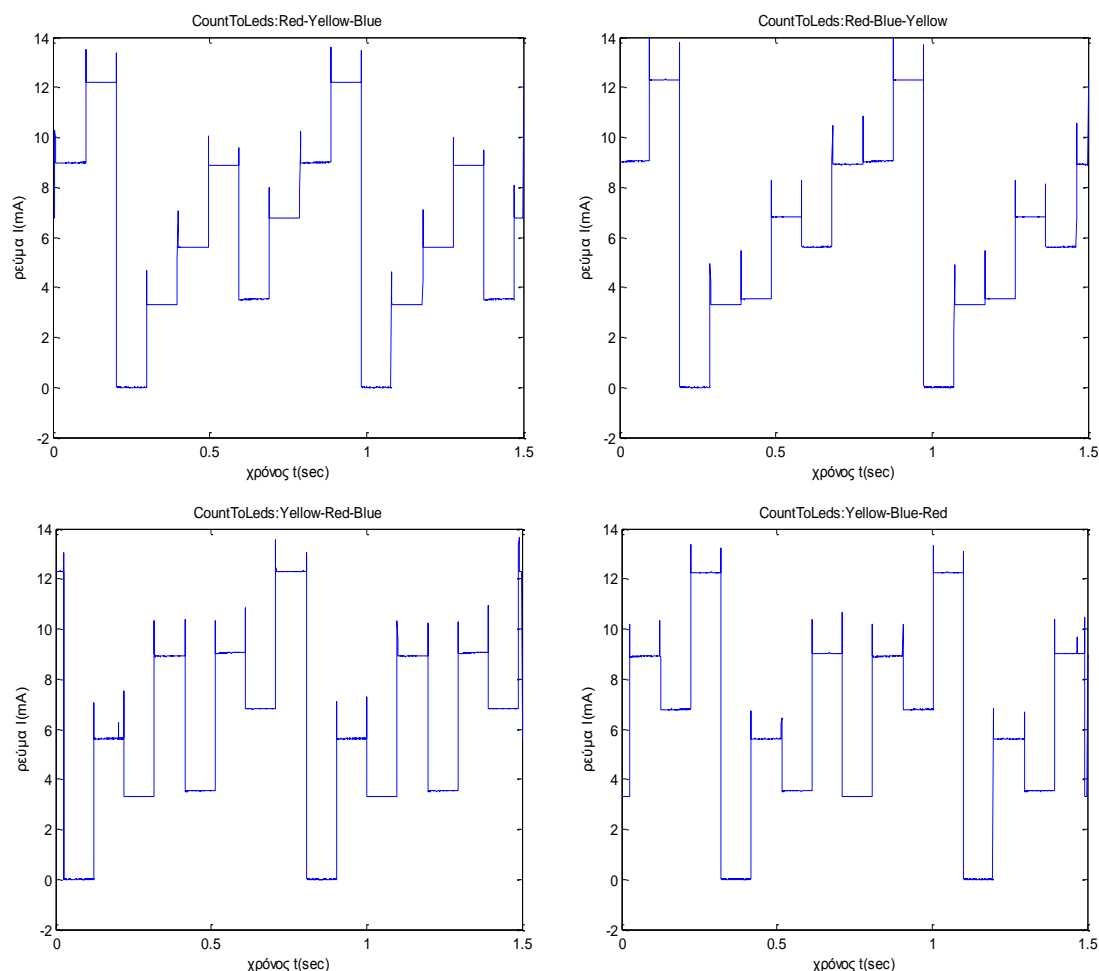
Σχήμα 62 Αποτελέσματα μετρήσεων ρευματικής κατανάλωσης εφαρμογής CountToLeds (TinyOS-2.x) μετρημένη μέσω της ηλεκτρονικής διάταξης με χρήση αντίστασης διακλάδωσης. Τα σχήματα αναπαριστούν διαφορετικούς συνδυασμούς ενεργοποίησης LEDs.
