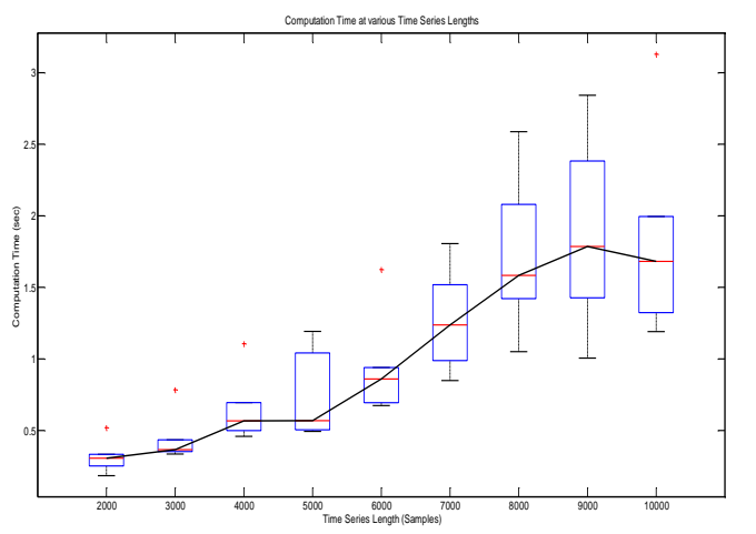
Σχήμα 103 Υπολογιστικός χρόνος για την ολοκλήρωση της Εμπειρικής Μεθόδου Αποσύνθεσης σε χρονοσειρές προερχόμενες από τη βάση MIT-BIH της Physionet. Το πρότυπο για την αύξηση του υπολογιστικού χρόνου με την αύξηση του πλήθους των δειγμάτων δεν είναι ομοιόμορφο για όλες τις χρονοσειρές καθώς και το εύρος του υπολογιστικού χρόνου για δεδομένο πλήθος δειγμάτων παρουσιάζει σημαντική διακύμανση. Στο σχήμα (β) παρουσιάζονται εκτενέστερες δοκιμές για σήματα από 2000-10000 δείγματα που προέρχονται από 46 διαφορετικά αρχεία της βάσης MIT-BIH της Physionet.
