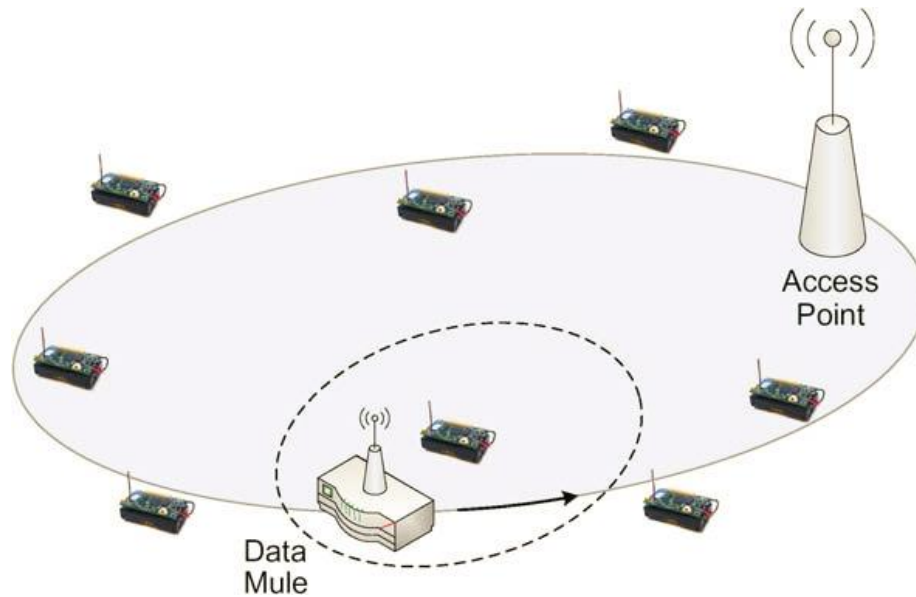
Σχήμα 11 Αρχιτεκτονική συστήματος ασύρματου δικτύου αισθητήρων με κινητούς αναμεταδότες
