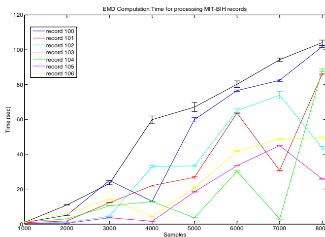
Σχήμα 103 Υπολογιστικός χρόνος για την ολοκλήρωση της Εμπειρικής Μεθόδου Αποσύνθεσης σε χρονοσειρές προερχόμενες από τη βάση MIT-BIH της Physionet. Το πρότυπο για την αύξηση του υπολογιστικού χρόνου με την αύξηση του πλήθους των δειγμάτων δεν είναι ομοιόμορφο για όλες τις χρονοσειρές καθώς και το εύρος του υπολογιστικού χρόνου για δεδομένο πλήθος δειγμάτων παρουσιάζει σημαντική διακύμανση. Στο σχήμα (β) παρουσιάζονται εκτενέστερες δοκιμές για σήματα από 2000-10000 δείγματα που προέρχονται από 46 διαφορετικά αρχεία της βάσης MIT-BIH της Physionet.
