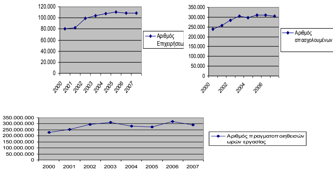
Σχήμα 6.4 : Εξέλιξη αριθμού επιχειρήσεων, απασχολούμενων και πραγματοποιηθεισών ωρών εργασίας στον κλάδο των κατασκευών, περιόδου 2000 – 2007
