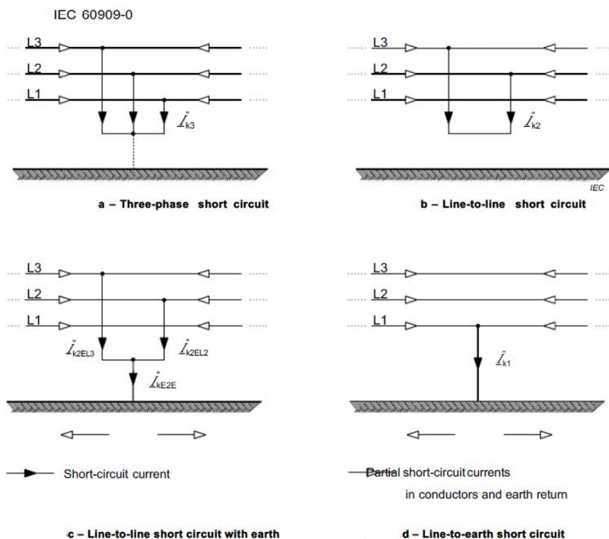
Σχήμα 8 Διάφοροι τύποι βραχυκυκλώματος
