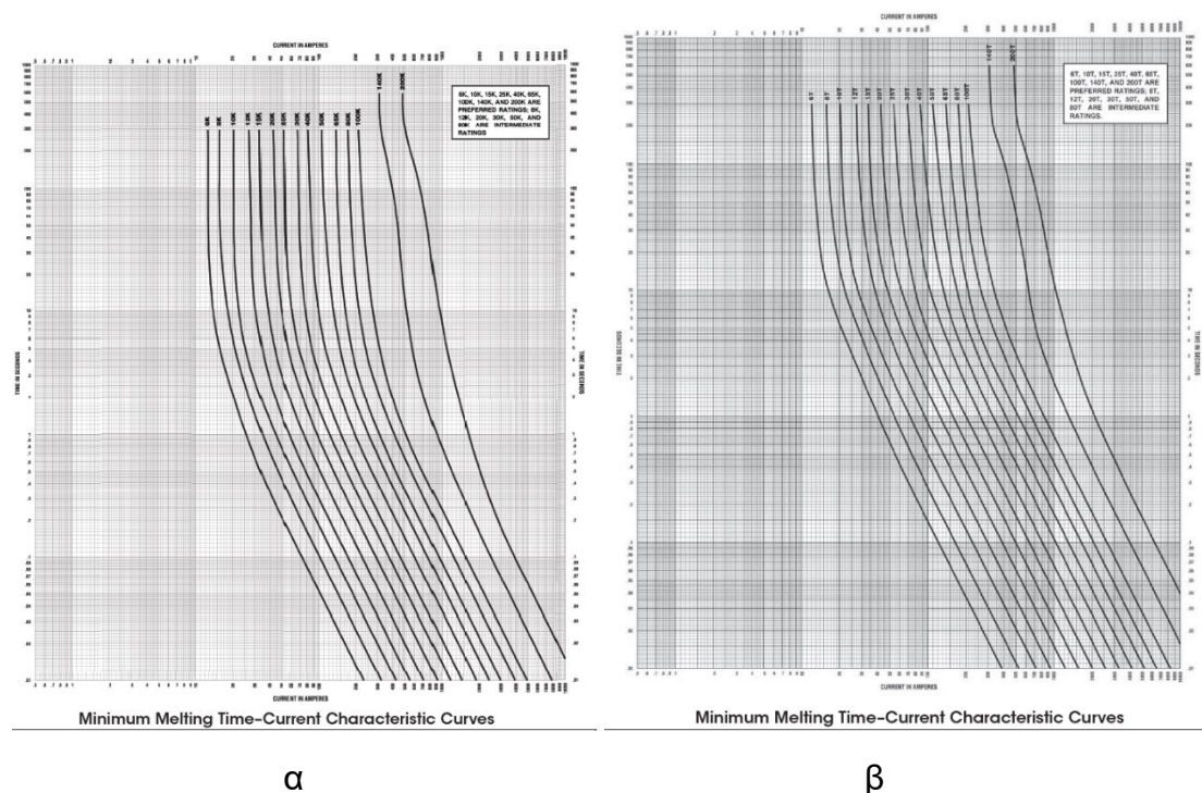
Σχήμα 5 Χαρακτηριστικές καμπύλες ρεύματος χρόνου Ασφαλειών Ταχείας και Βραδείας τήξης
