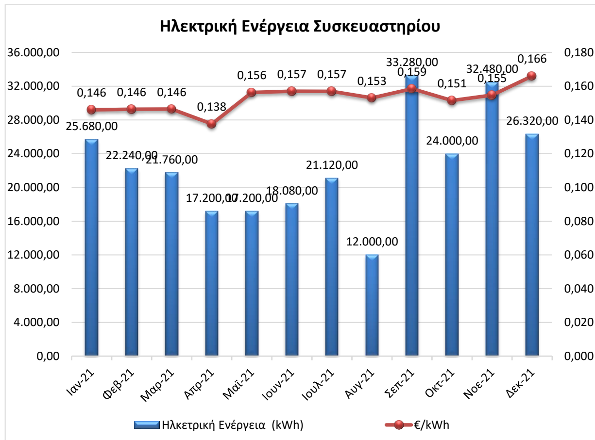
Διάγραμμα 13: Διάγραμμα ηλεκτρικής ενέργειας εγκατάστασης
