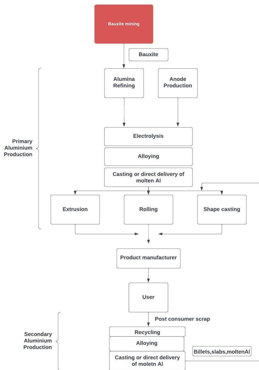
Εικόνα 1: Διαγραμματική απεικόνιση της διαδικασίας παραγωγής του αλουμινίου (Brough & Jouhara, 2020, ίδια επεξεργασία)
