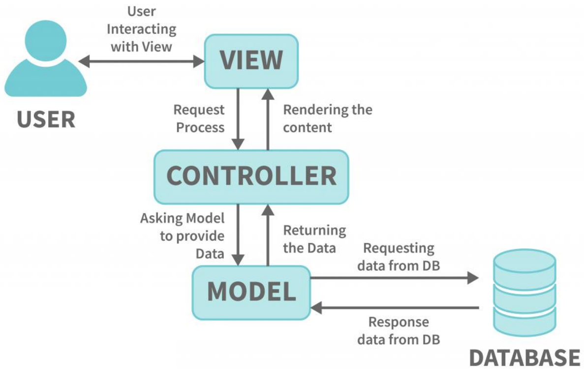
Εικόνα 2.1.1: Διάγραμμα λειτουργία MVC Αρχιτεκτονικής [35]
