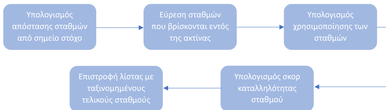
Εικόνα 4.1.1: Διάγραμμα ροής αλγορίθμου βελτιστοποίησης
