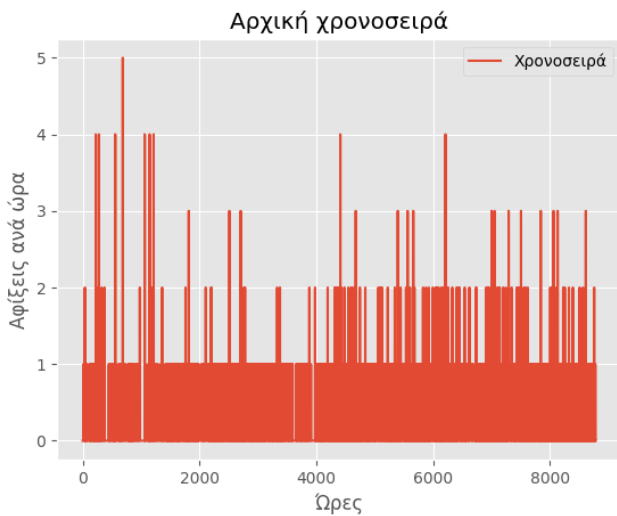
Εικόνα 3.2.1.1: Αρχική χρονοσειρά αφίξεων κατηγορίας 1
