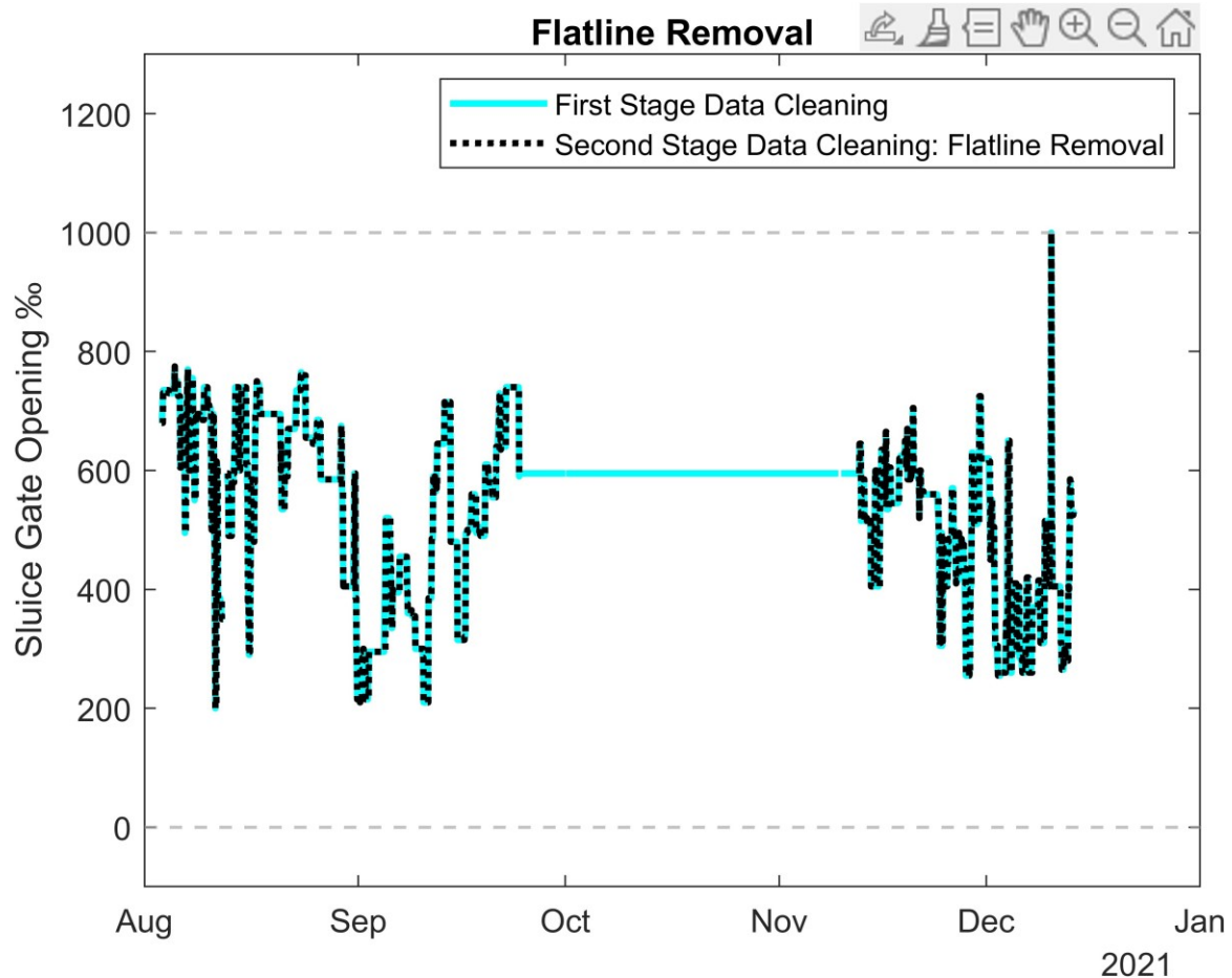
Γράφημα 6.7: Γραφική παράσταση χρονοσειράς ανοίγματος δεξιού θυροφράγματος με ταυτόχρονη αναπαράσταση αποτελέσματος πρώτου και δεύτερου σταδίου καθαρίσματος δεδομένων. Το δεύτερο στάδιο δεν περιλαμβάνει τμήματα με ισοπέδωση σήματος.
