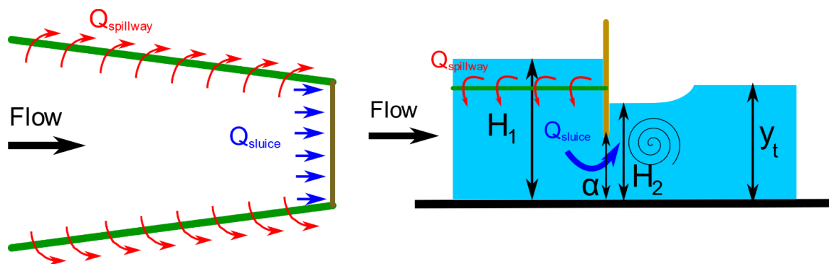
Σχήμα 4.2: Κάτοψη και τομή διάταξης τύπου \Lambda
