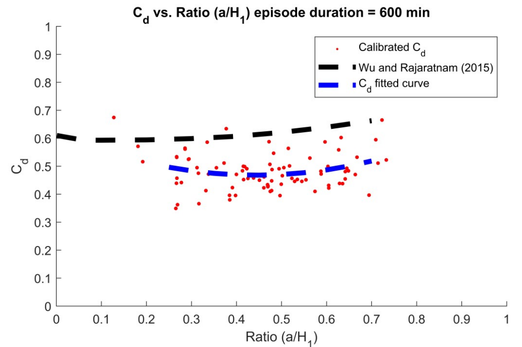
Γράφημα 7.8: Νέφος τιμών C_d συναρτήσει του λόγου a/H_1 για επεισόδια \geq 10 hr
