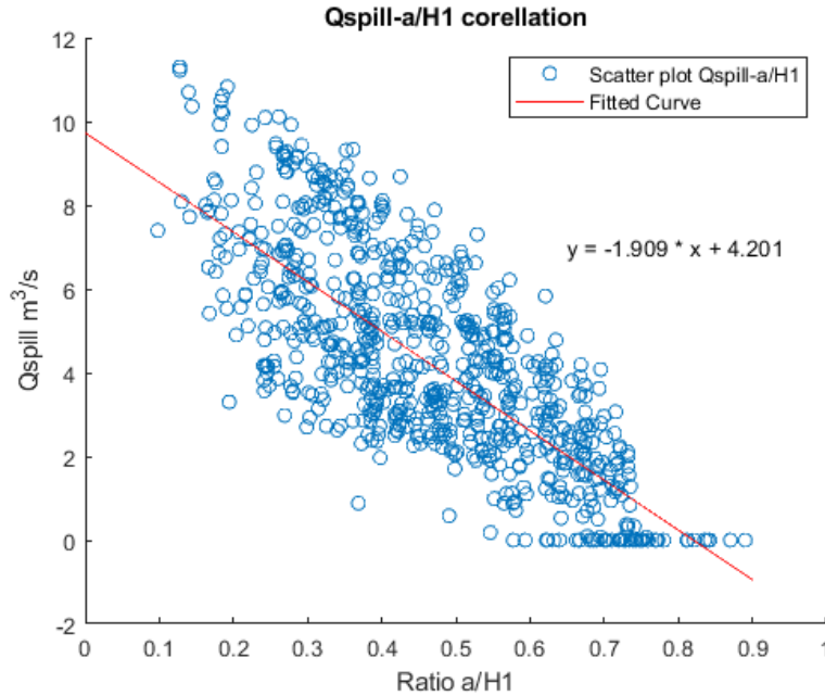
Γράφημα 7.9: Συσχέτιση παροχής υπερχειλίσης συγκριτικά με το λόγο a/H_1
