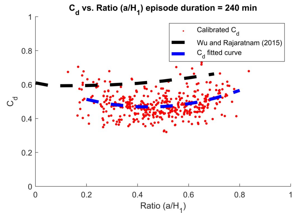
Γράφημα 7.6: Νέφος τιμών C_d συναρτήσει του λόγου a/H_1 για επεισόδια \geq 4 hr
