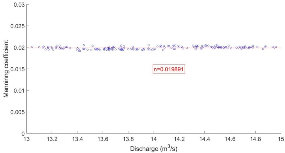
Σχήμα 5.1 Βαθμονομημένος συντελεστής τραχύτητας για διάφορες παροχές.
