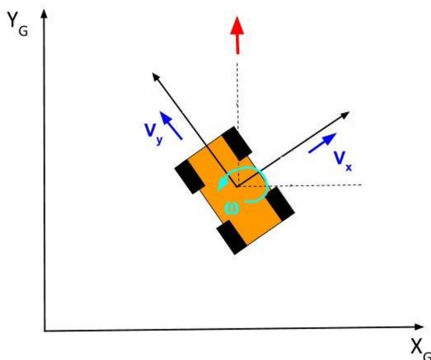
Σχήμα 4-22. Παράσταση των συνιστωσών γραμμικής και γωνιακής ταχύτητας με τις οποίες μπορεί να κινηθεί το ρομπότ.
