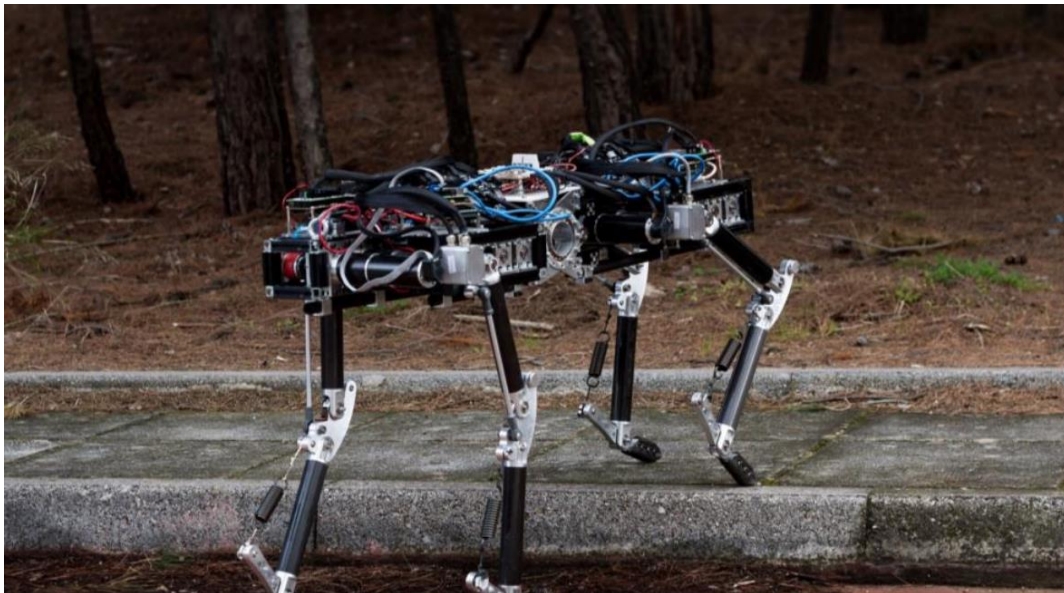
Σχήμα 2-1. Το τετράποδο ρομπότ Laelaps.
