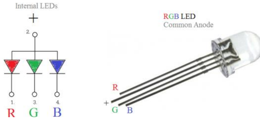
Εικόνα 41: Φωτοдиодος κοινής ανόδου
