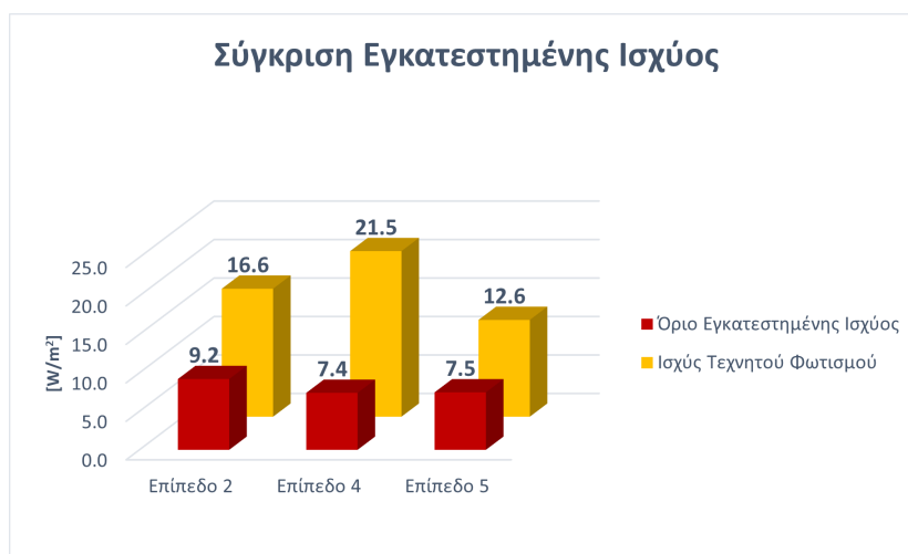
Σχήμα 42: Σύγκριση υφιστάμενης εγκατάστασης με όρια Τ.Ο.Τ.Ε.Ε.
