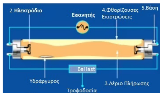
Σχήμα 1: Αναπαράσταση δομής και συνδεσμολογίας λαμπτήρα φθορισμού.
