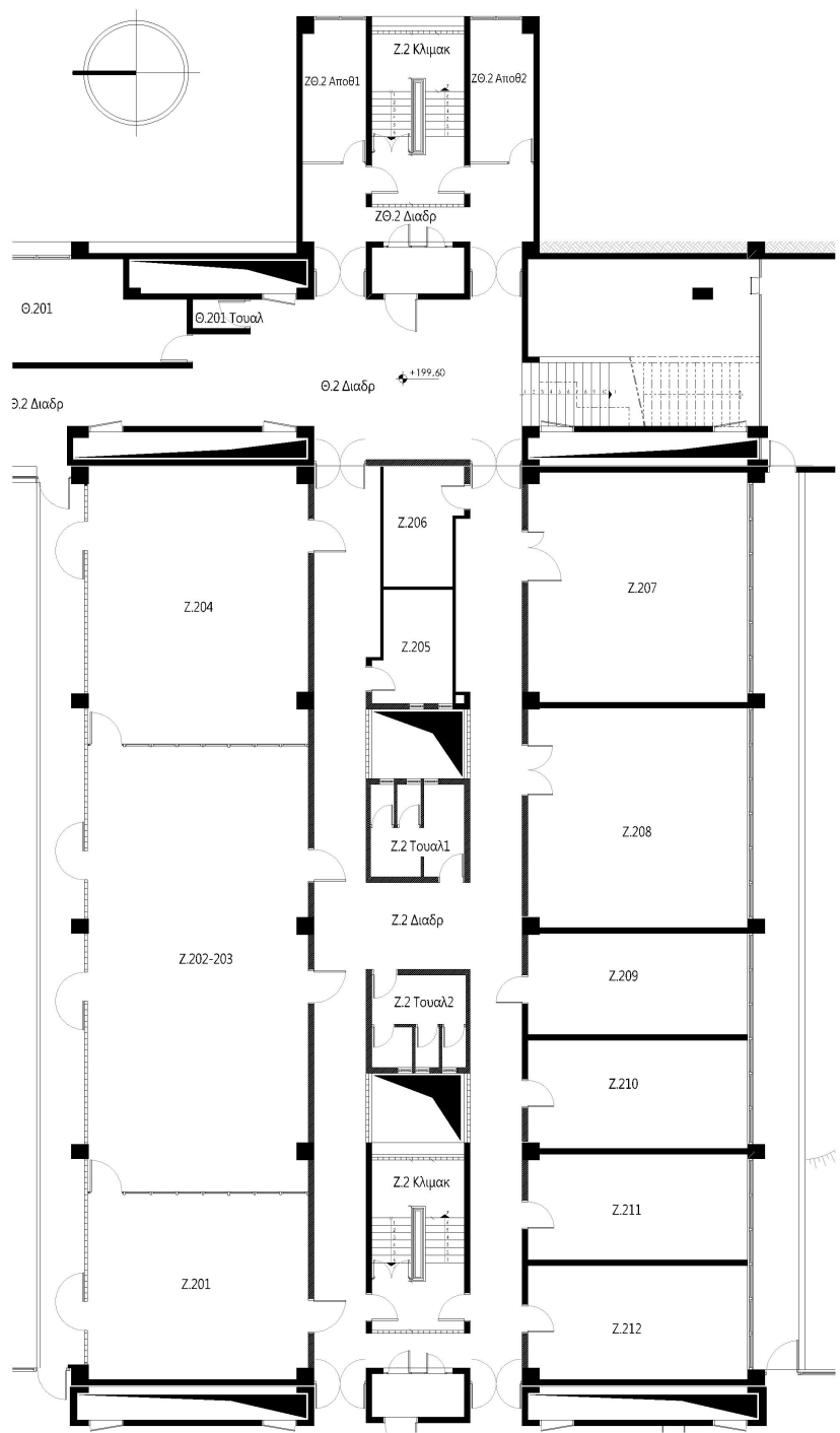
Σχήμα 17: Κάτοψη πτέρυγες Z-ZΘ του επιπέδου 2
