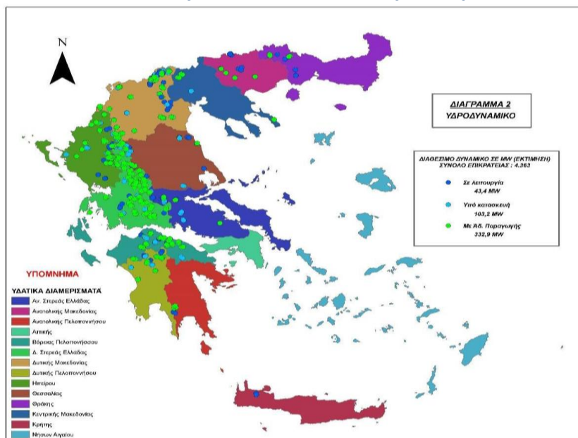
Χάρτης 13: Υδροδυναμικό της χώρας
