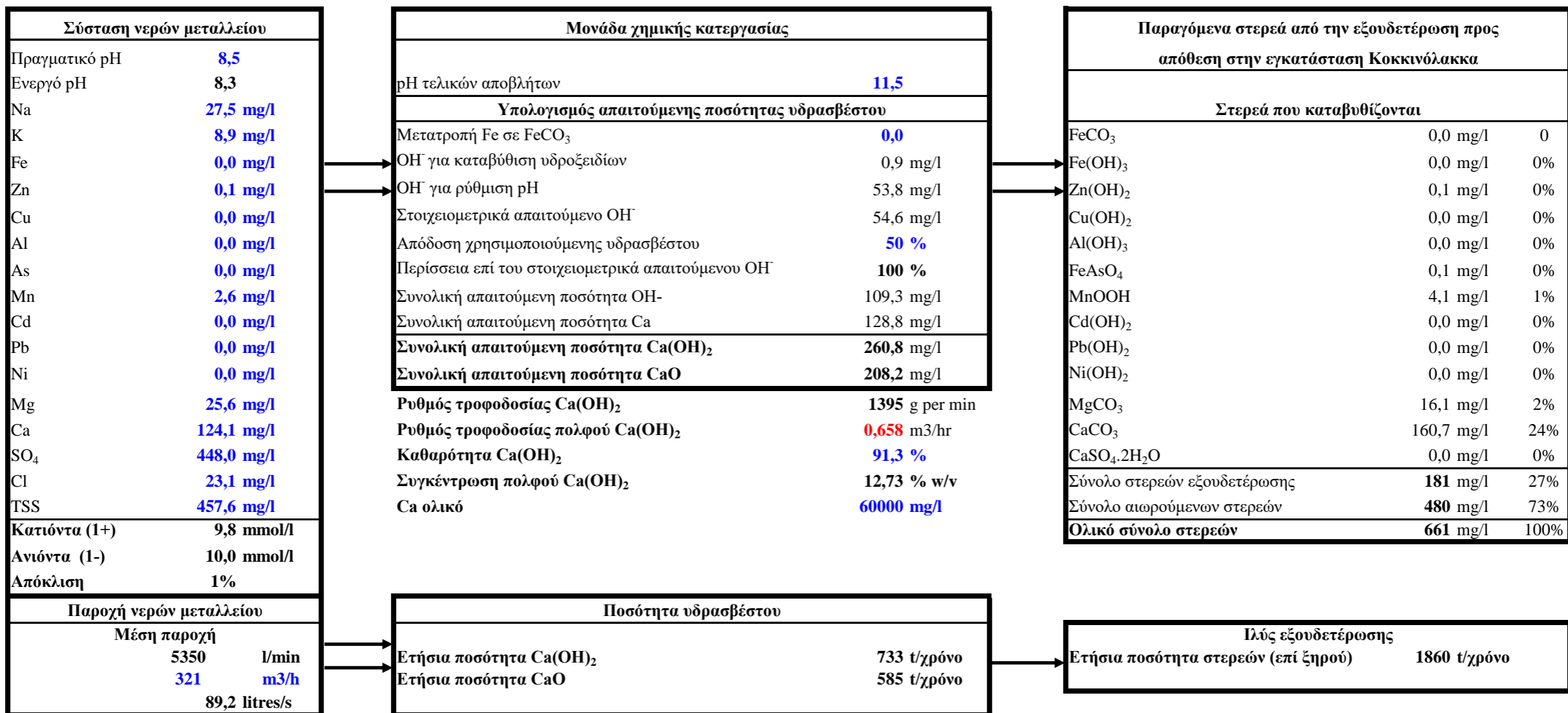
Πίνακας V.4: Προσομοίωση της μονάδας εξουδετέρωσης νερών μεταλλείου Μαύρων Πετρών (Στοιχεία παρακολούθησης 2012 – 2021)
