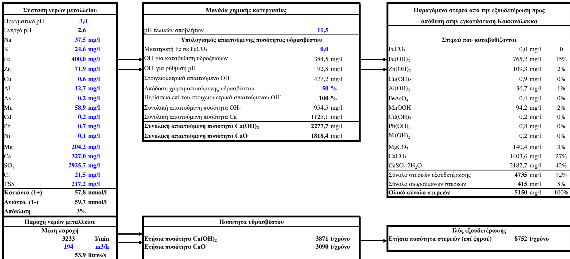
Πίνακας V.6: Προσομοίωση της μονάδας εξουδετέρωσης νερών μεταλλείου Μαντέμ Λάκκου (Στοιχεία παρακολούθησης 1997 – 2021)
