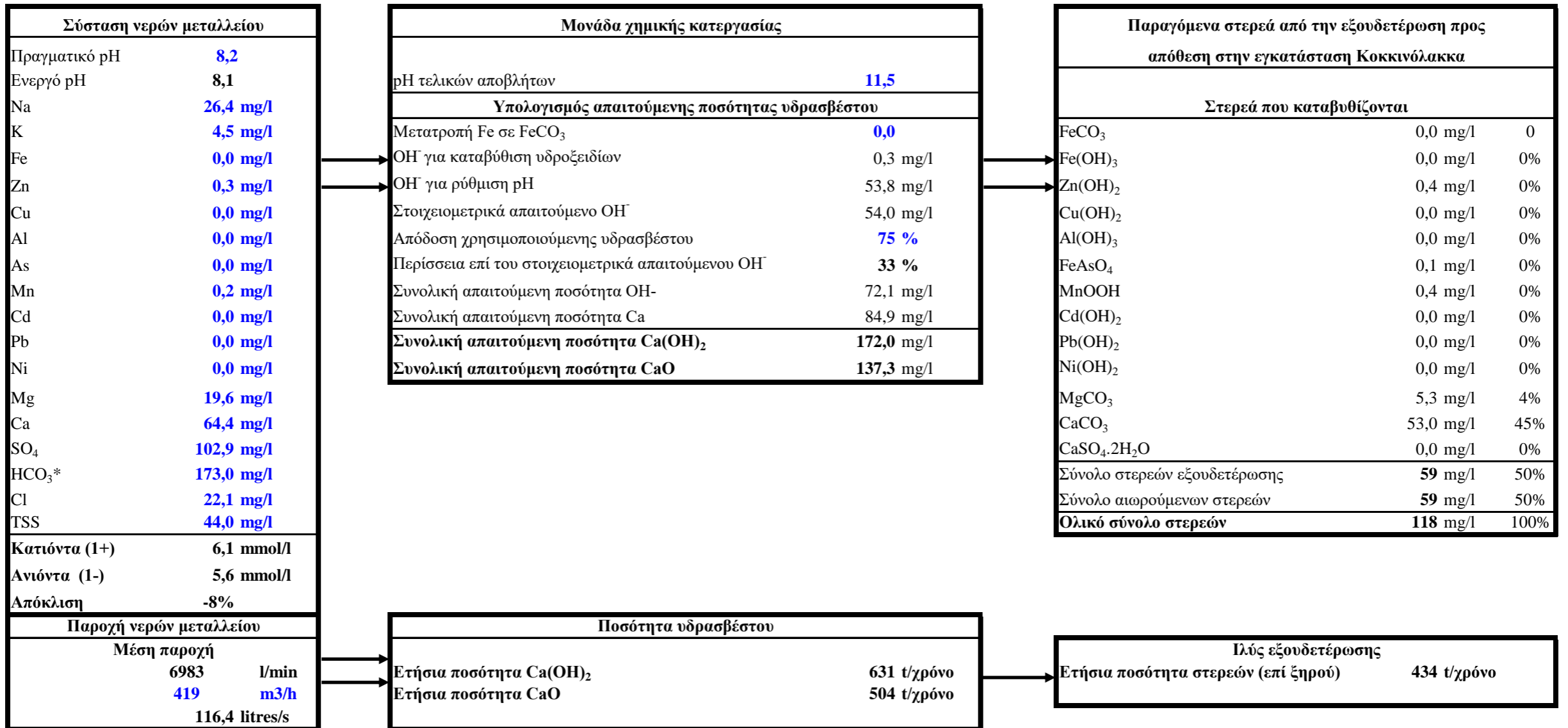
Πίνακας V.2: Προσομοίωση της μονάδας εξουδετέρωσης νερών μεταλλείου Ολυμπιάδας (Στοιχεία παρακολούθησης 1996 – 2021)
