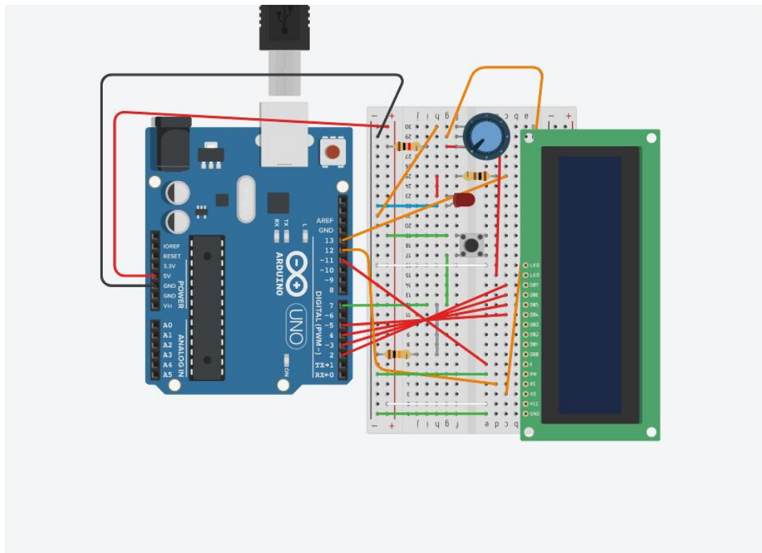
Εικόνα 23: Ενδιάμεσο κύκλωμα
