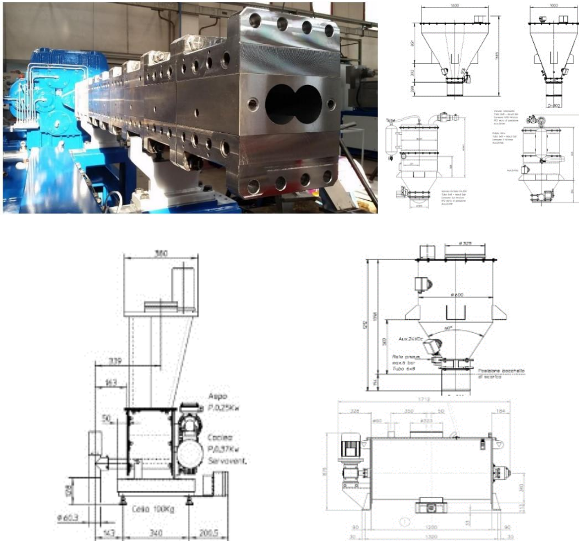
Εικόνα 18: Τεχνικά Χαρακτηριστικά Μηχανήματος Γραμμής Παραγωγής
