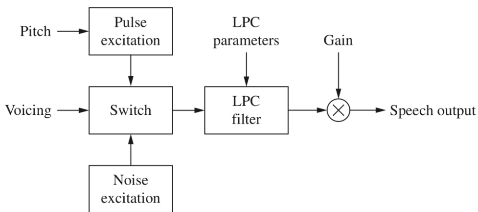
Σχήμα 5.9 Αποκωδικοποιητής LPC.[15]
