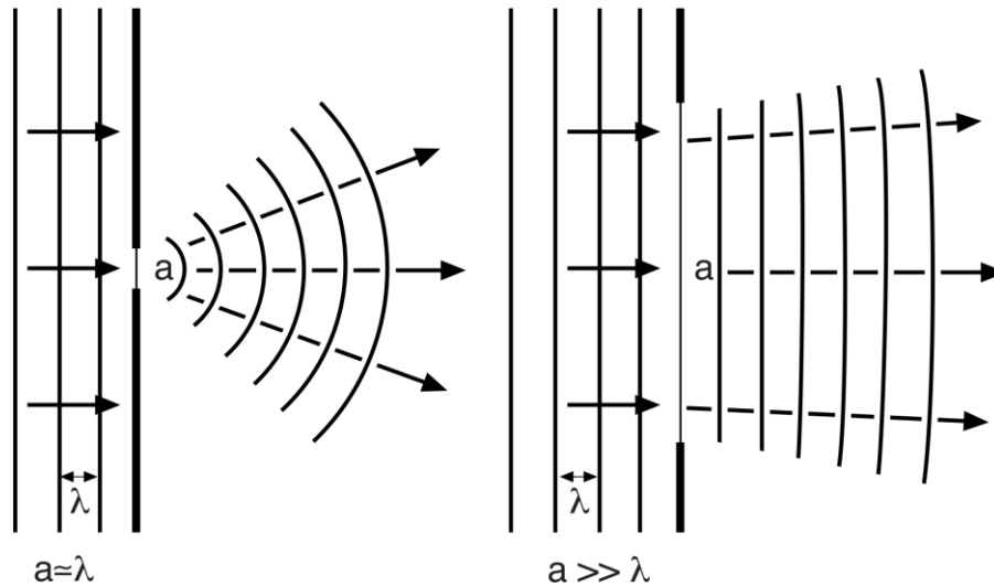
Σχήμα 3.9 Περίθλαση κύματος που συναντά εμπόδιο με οπή, το μέγεθος της οποίας συγκρίνεται με το μήκος κύματός του (αριστερά), ή είναι πολύ μεγαλύτερο αυτού (δεξιά).[9]
