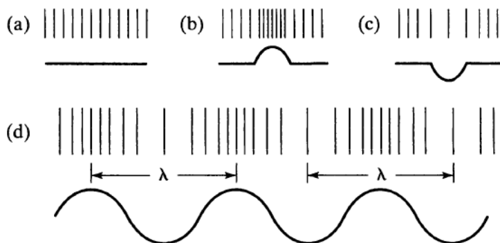
Σχήμα 3.6 Εγκάρσια αναπαράσταση (a) χορδής σε ισορροπία, (b) πύκνωσης, (c) αραιώσης, και (d) σειράς πυκνώσεων και αραιώσεων.[10]
