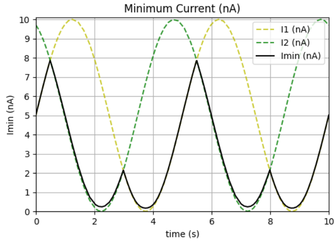
Σχήμα 4.8: Η min έξοδος του κυκλώματος MIN-MAX με δύο ημιτονειδή ρεύματα εισόδου πλάτους 10\text{nA} και διαφοράς φάσης 110\text{ deg} .
