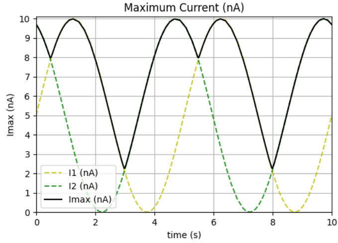
Σχήμα 4.7: Η max έξοδος του κυκλώματος MIN-MAX με δύο ημιτονειδή ρεύματα εισόδου πλάτους 10\text{nA} και διαφοράς φάσης 110\text{ deg} .
