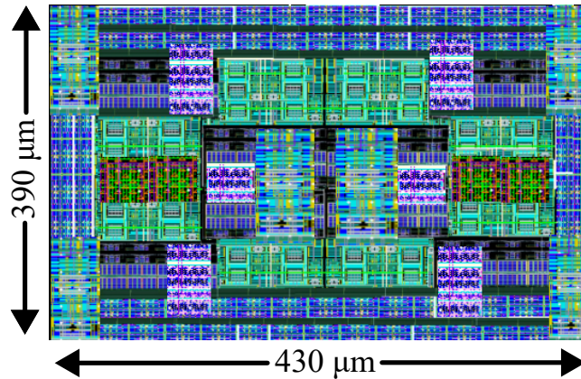
Σχήμα 5.1: Η υλοποίηση της διάταξης του προτεινόμενου αναλογικού ασαφούς ελεγκτή στην τεχνολογία TSMC 90nm.
