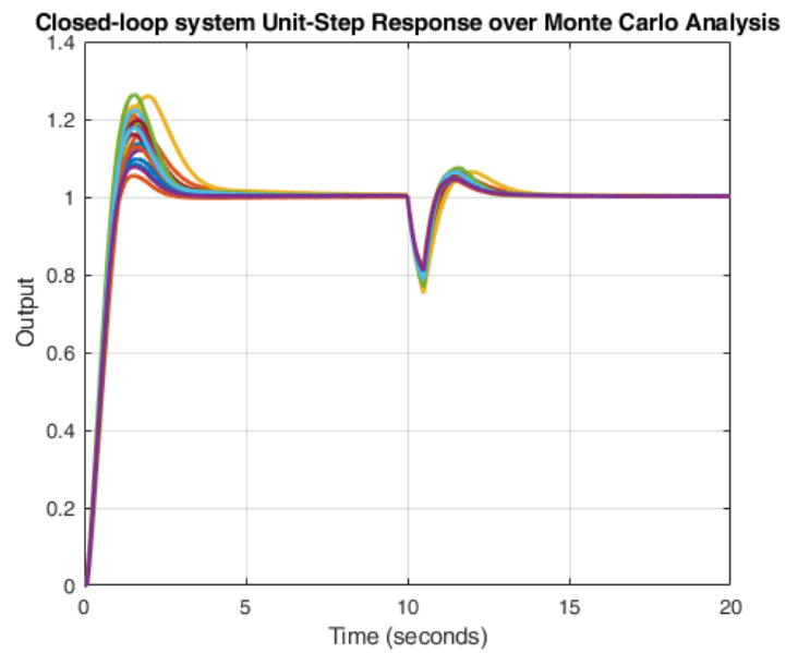
Σχήμα 5.4: Η βηματική απόκριση της υλοποίησης υλικού του συστήματος κλειστού βρόχου για ανάλυση Μοντε Κάρλο με N = 100 σημεία για να δοκιμαστεί η ανθεκτικότητα του κυκλώματος.
