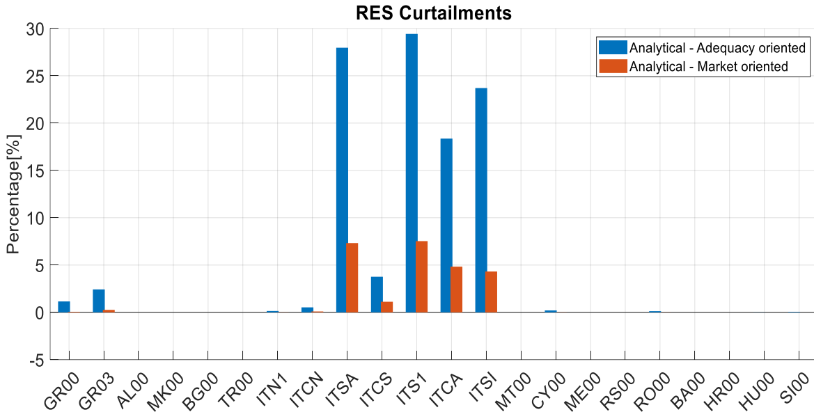
Σχήμα 32 : Περικοπές ΑΠΕ
