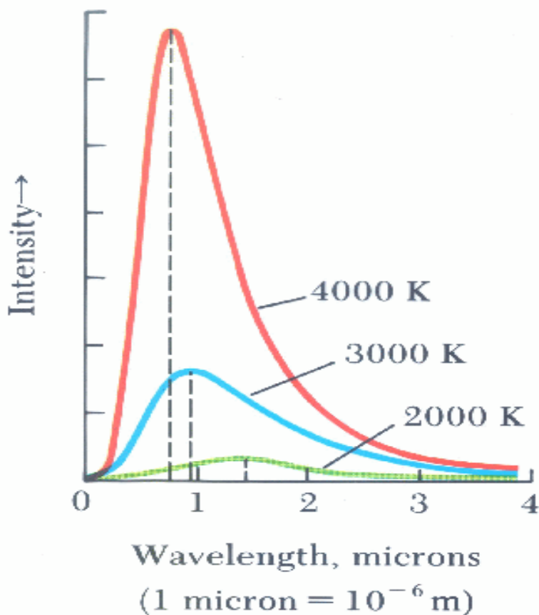
Σχήμα : Ένταση της ακτινοβολίας που εκπέμπεται από μέλαν σώμα ως συνάρτηση της συχνότητας και της θερμοκρασίας.
