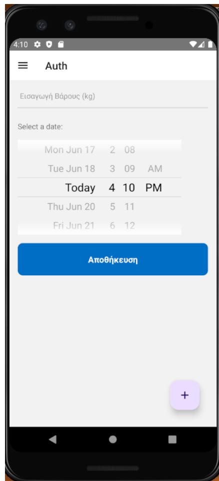
Σχήμα 6.8: Εισαγωγή Βάρους
