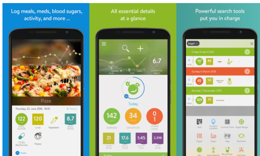
Σχήμα 3.9: Mysugr App
