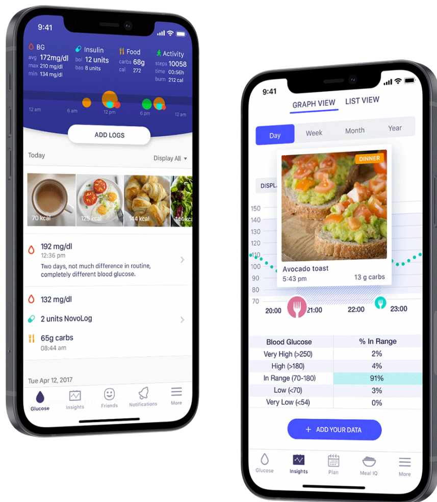
Σχήμα 3.10: GlucoseBuddy App
