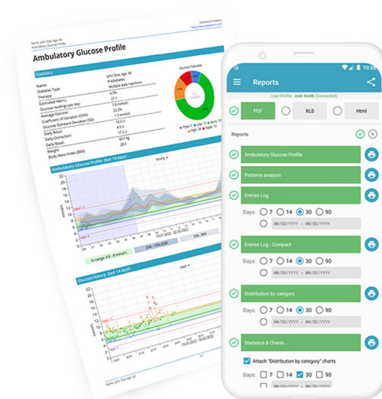
Σχήμα 3.11: Diabetes:M Platform
