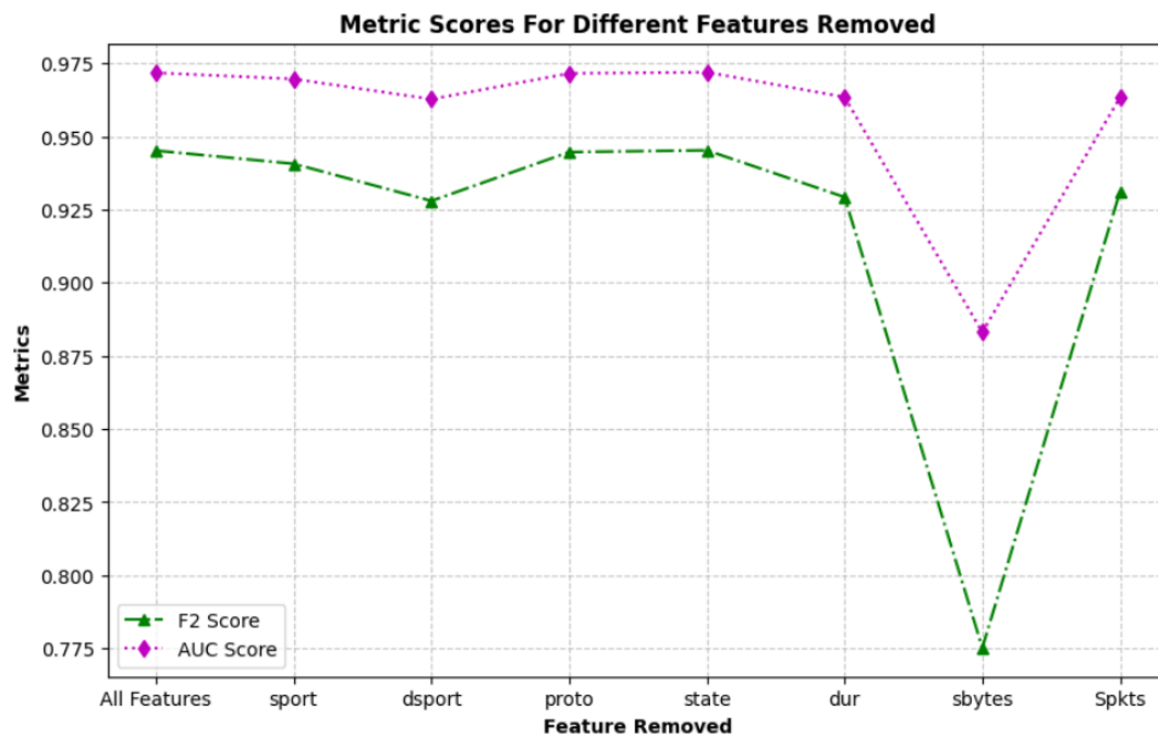
Σχήμα 3..5.1.1: Απόδοση Μετρικών με την αφαίρεση ενός πρώτου χαρακτηριστικού
