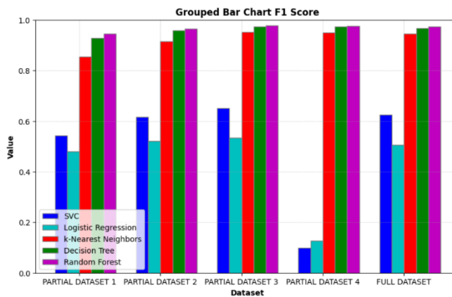
Σχήμα 3.2.6.7: Απόδοση Μετρικής F1 Score σε όλες τις πειραματικές διαδικασίες
