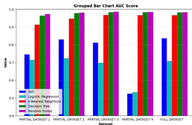
Σχήμα 3.2.6.9: Απόδοση Μετρικής AUC Score σε όλες τις πειραματικές διαδικασίες
