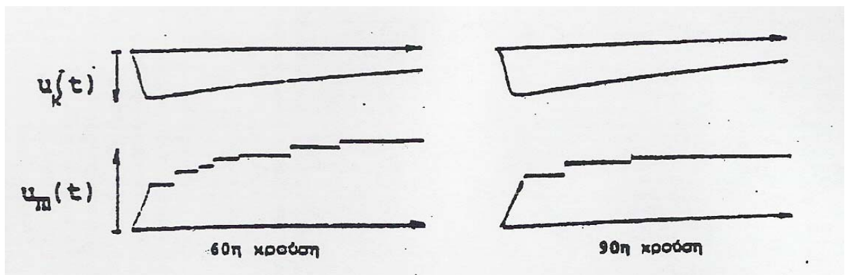
Σχήμα 5.2-4 : Άλματα δυναμικού κατά την 60η και 90η κρούση σε μονωτικό υλικό pertinax πάχους 2mm.
