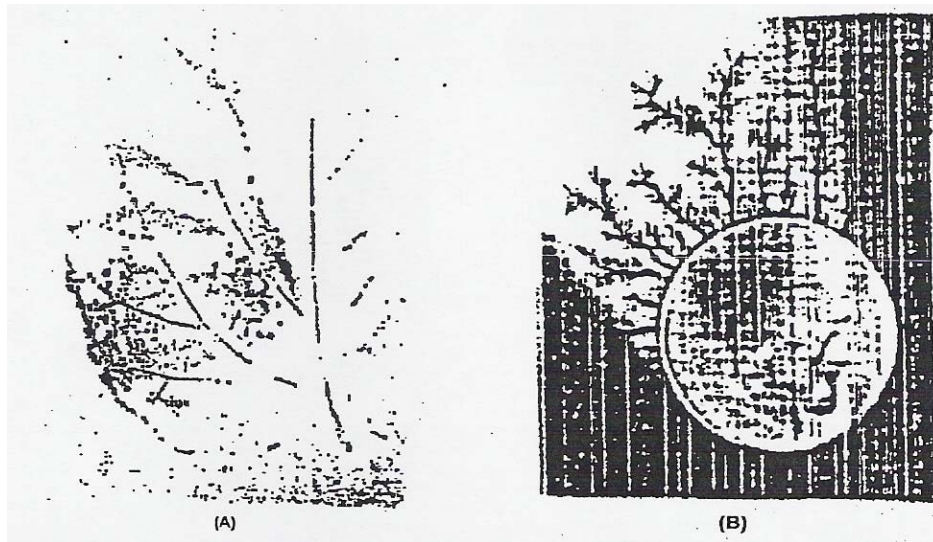
Σχήμα 5.5-2 : Προσβολή του φωτογραφικού φιλμ κατά την καταπόνηση στερεού μονωτικού πλησίον της περιοχής τιμών για την επιφανειακή διάσπαση στον αέρα, υπό κρουστική τάση 1,2/50 μs. (A) Φύλλο δέντρου (B) Μεταλλικό κέρμα
