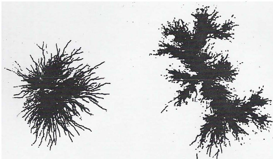
Σχήμα 5.5-3 : Φωτογραφίες δενδριτών κατά την καταπόνηση στερεού μονωτικού στο αέρα υπό κρουστική τάση 1,2/50 μs. (A) : Δενδρίτης σε τιμές πεδίου πλησίον της περιοχής τιμών για την επιφανειακή διάσπαση. (B) : Δενδρίτης κατά την επιφανειακή διάσπαση.
