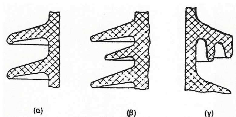
Σχήμα 1.9-1 : Κατανομές τυπικών κεραμικών μονωτήρων με πλευρικές προεξοχές.
