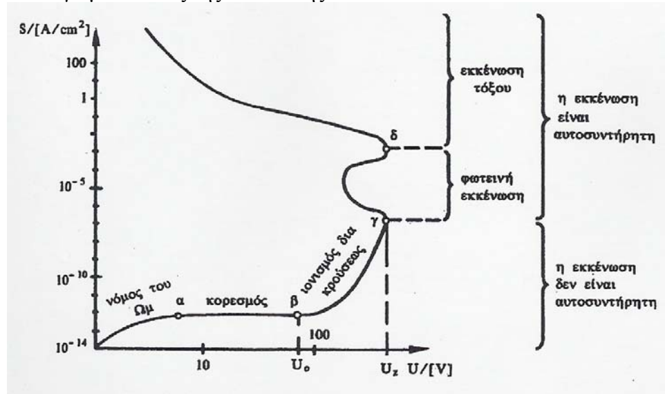
Σχήμα 4.11-1 : Χαρακτηριστική "τάσης - πυκνότητας ροής" ενός αερίου υπό κανονικές συνθήκες κατά G. Orberdorffer.
