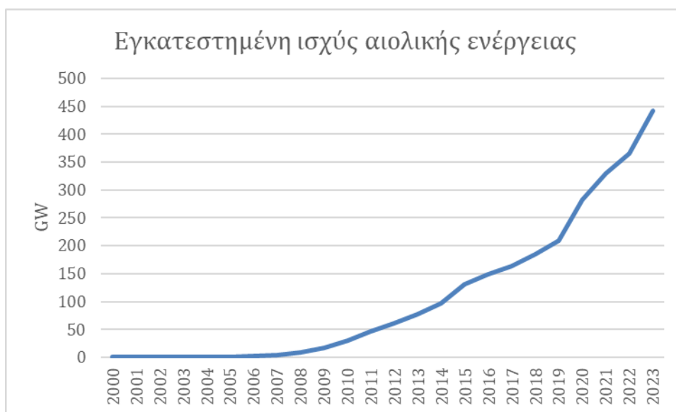
Εικόνα 33: Η εγκατεστημένη ισχύς αιολικής ενέργειας της Κίνας
