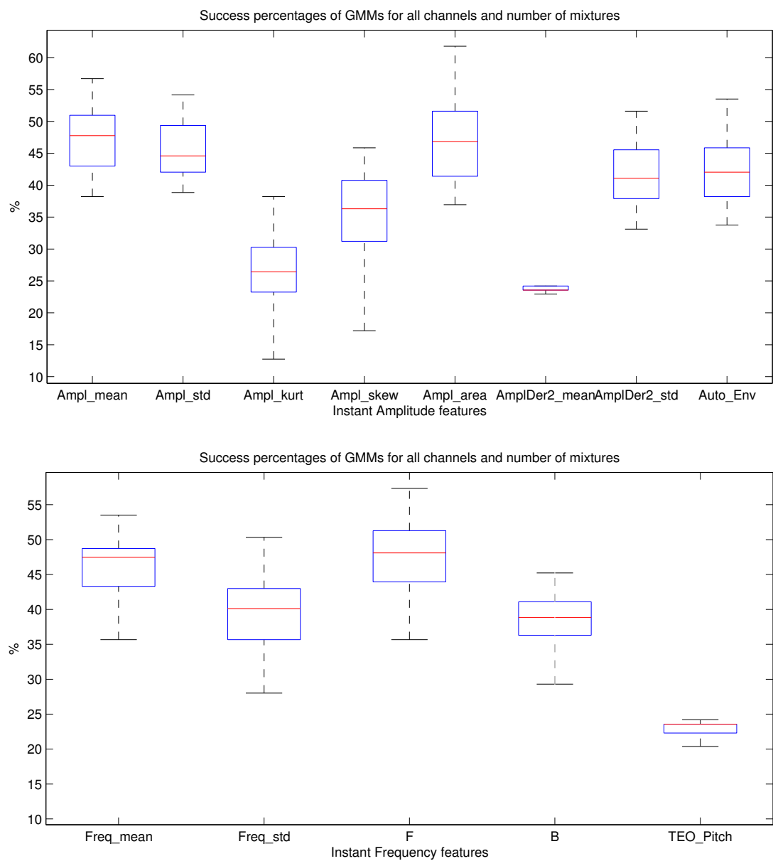
Σχήμα 7.2: Μέση τιμή ποσοστών επιτυχίας GMMs για όλα τα χαρακτηριστικά.
