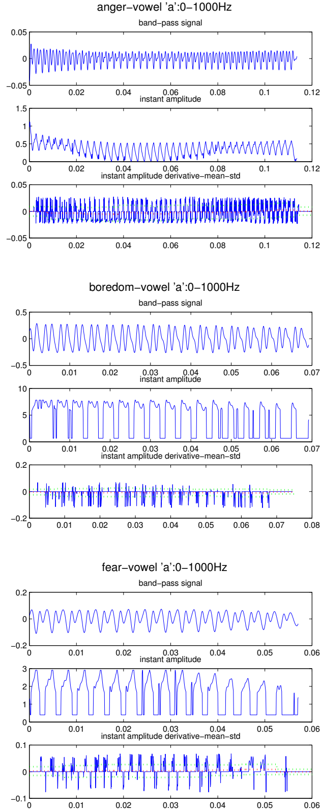
Σχήμα 5.5: Γραφική απεικόνιση του ζωνοπερατού σήματος του φωνήεντος 'a', , του στιγμιαίου πλάτους και της παραγώγου του στο θυμό, την πλήξη και το φόβο. Η κόκκινη διακεκομμένη γραμμή απεικονίζει το μέσο όρο σε κάθε frame και οι δύο πράσινες διακεκομμένες δείχνουν την απόσταση της τυπικής απόκλισης από το μέσο όρο.
