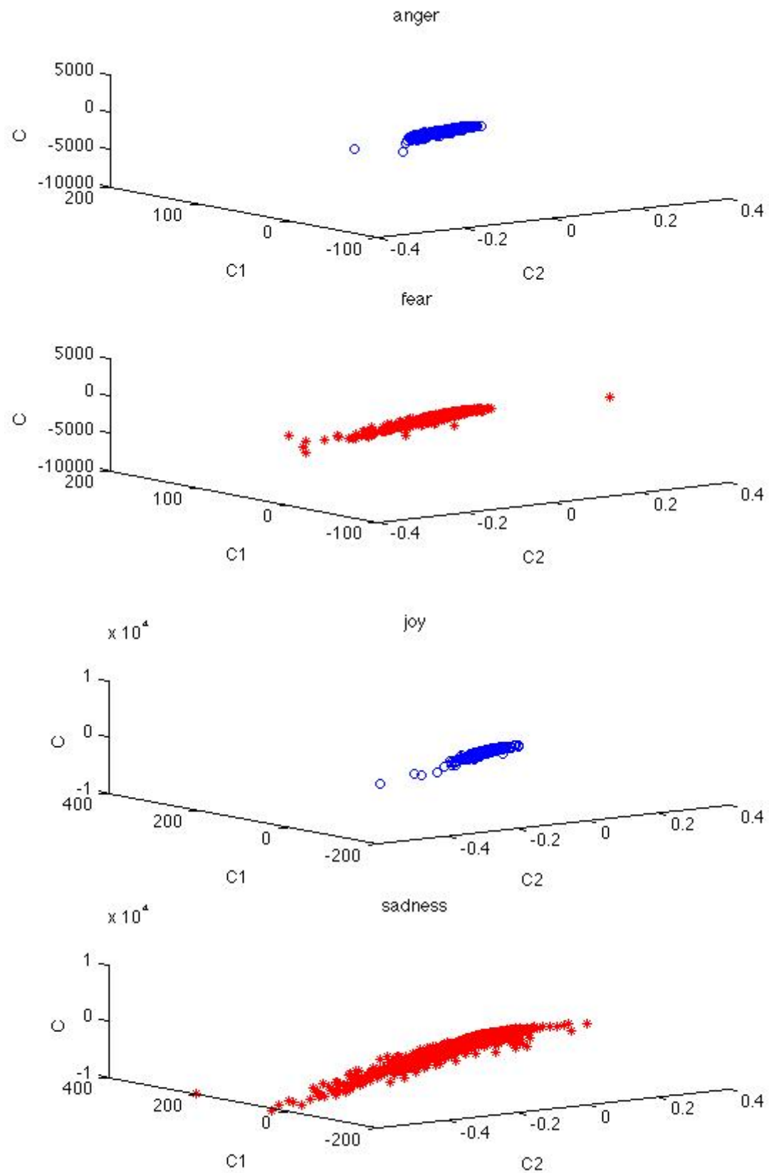
Σχήμα 5.20: Τρισδιάστατη αναπαράσταση των συντελεστών C_0 , C_1 και C_2 του πολυωνύμου p(X) για τα ζευγάρια συναισθημάτων θυμός - φόβος και χαρά - λύπη
