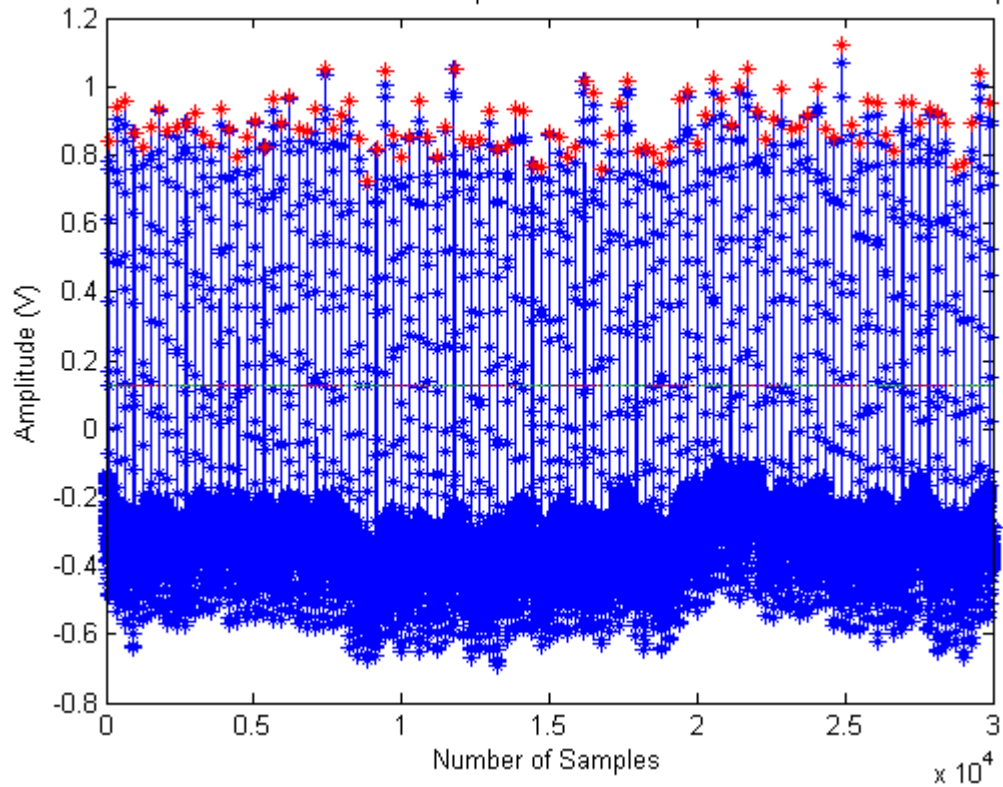
Εικόνα 63 Σήμα 100: Τα δείγματα φαίνονται με μπλε αστερίσκο, τα ανιχνευμένα peaks με κόκκινο και το κατώφλι με την μαύρη γραμμή
