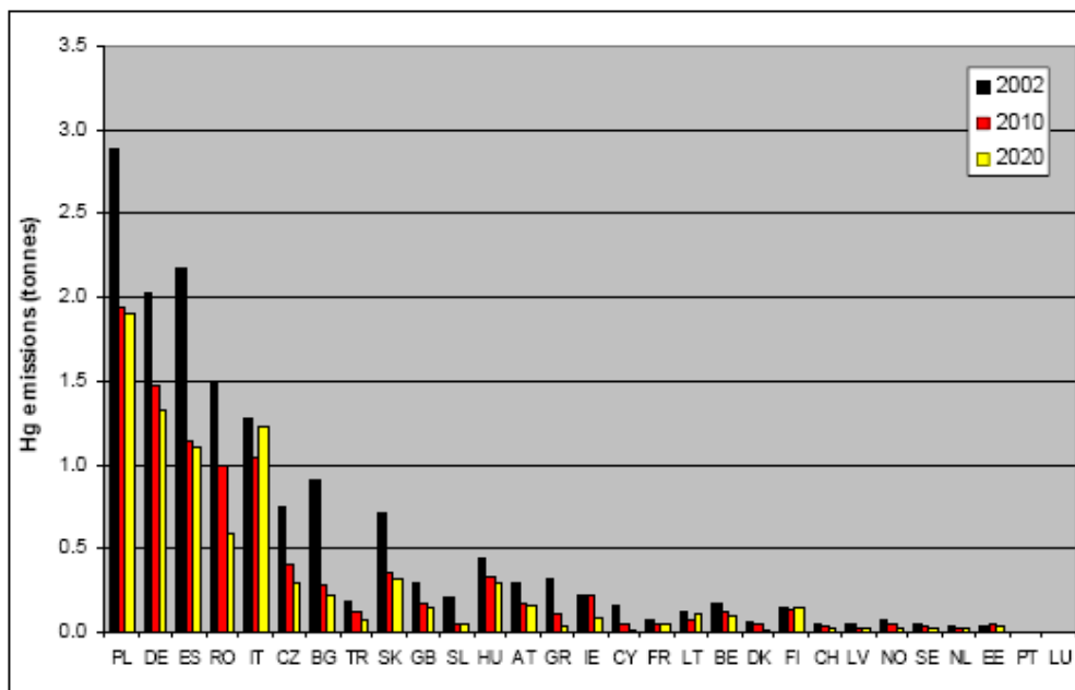
Σχήμα 4.18: Απεικόνιση των βιομηχανικών SCI εκπομπών (από στερεά καύσιμα) για τα έτη 2010 και 2020 σε σύγκριση με τον τωρινό κατάλογο εκπομπών
