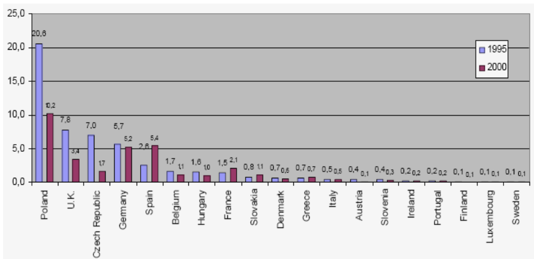
Σχήμα 2.9: Υδράργυρος (τόνοι/έτος) από την καύση άνθρακα στις εγκαταστάσεις παραγωγής ενέργειας πάνω από 50MWth
