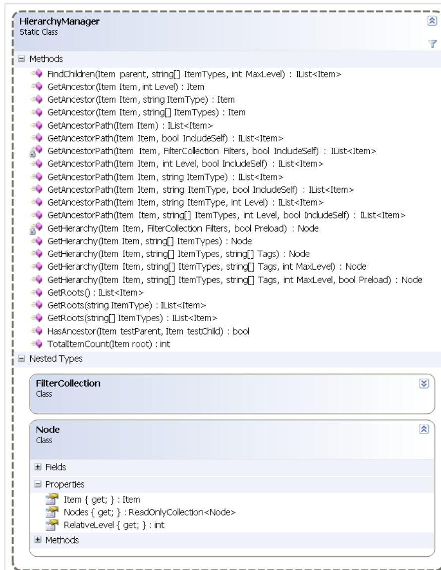
Εικόνα 5-5 Διάγραμμα κλάσης του HierarchyManager
