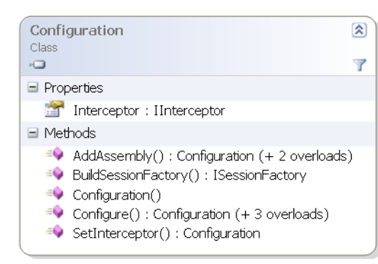
Εικόνα 3-9 Διάγραμμα κλάσης του Configuration
