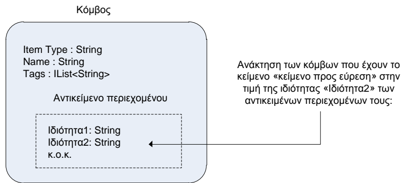
Εικόνα 4-19 Ανάκτηση κόμβων βάσει ενός δοσμένου κειμένου
