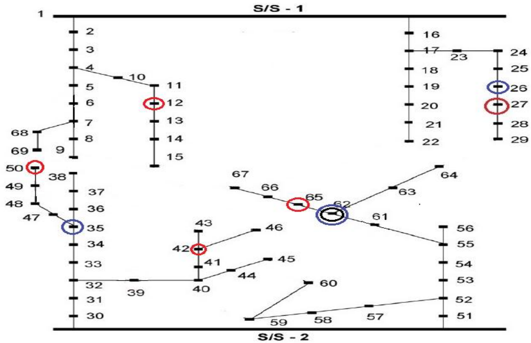
Σχήμα 4.3: Τοποθέτηση ΜΔΠ με βάση τις απώλειες και τη διακύμανση της τάσης, μετά τη διείσδυση των ηλεκτρικών οχημάτων
