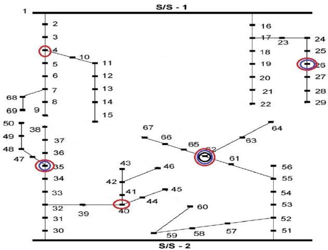
Σχήμα 4.5: Τοποθέτηση ΜΔΠ με βάση οικονομικά κίνητρα, μετά τη διεξόδου των ηλεκτρικών οχημάτων με ομοιόμορφη φόρτιση
