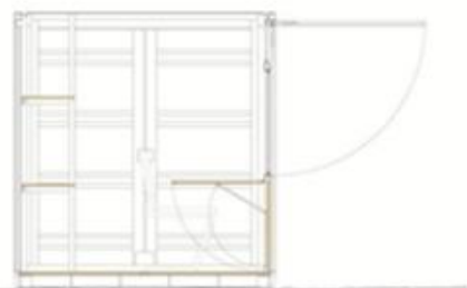
Τομή Αποθήκη οπτικοακουστικών μέσων / Εργαστήριο
