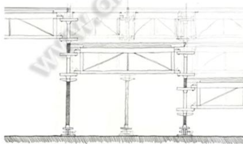
Όψη κερκίδων
