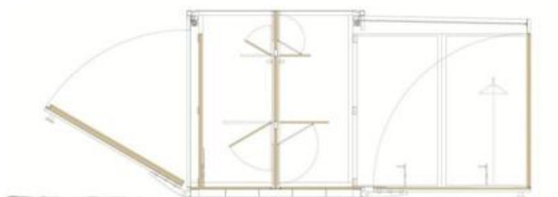
Τομή ανοικτή - καμαρίνια
