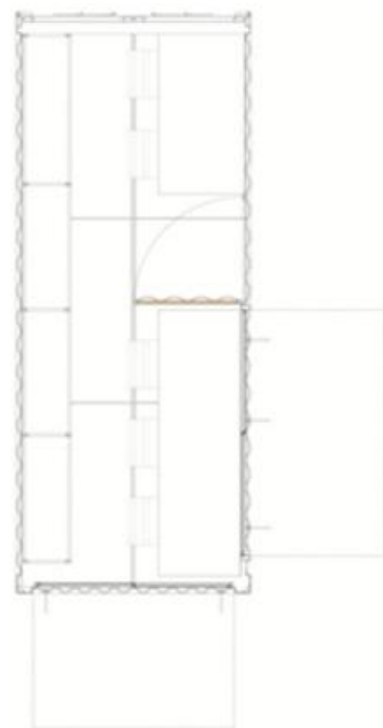
Κάτοψη Αποθήκη οπτικοακουστικών μέσων / Εργαστήριο
