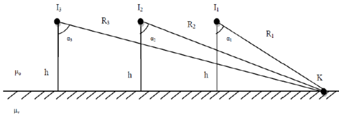
Σχήμα 5.2 Υπολογισμός του μαγνητικού πεδίου τριών αγωγών, σε σημείο Κ που απέχει από αυτούς απόσταση R. I_1, I_2, I_3 : ένταση ρεύματος αγωγών \mu_0 : μαγνητική διαπερατότητα του κενού \mu_\gamma : μαγνητική διαπερατότητα του εδάφους
