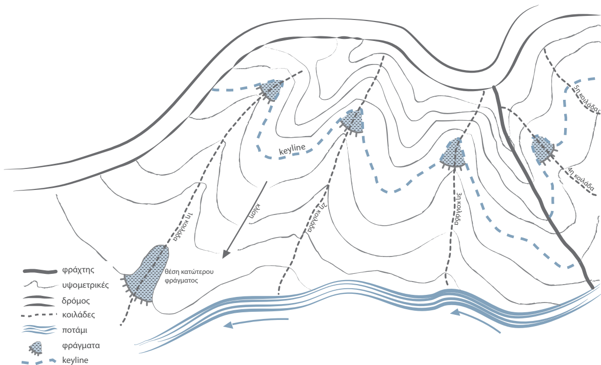
εικ. 8: σκίτσο εφαρμογής του keyline design για τη συλλογή νερού. πηγή: 'The Keyline Plan', P.A. Yeomans. Ιδία επεξεργασία
