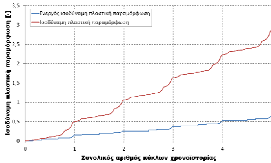
Σύγκριση πλαστικών παραμορφώσεων IPE 355s_03
