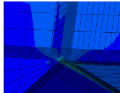
Αρχή ενεργού βλάβης IPE 355s_02
