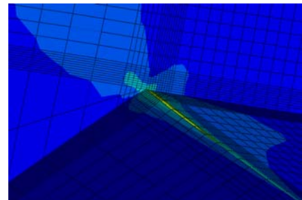
Αρχή ενεργού βλάβης IPE 355s_04
