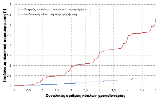
Σύγκριση πλαστικών παραμορφώσεων IPE 355s_03
