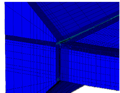
Σύγκριση πλαστικών παραμορφώσεων IPE 355s_03
