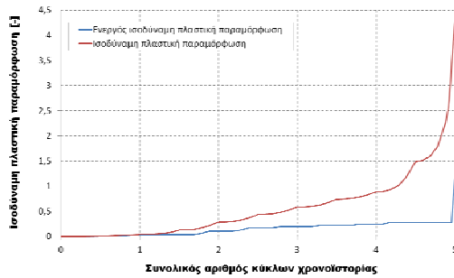
Σύγκριση πλαστικών παραμορφώσεων IPE 355ns_02
