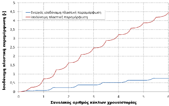
Σύγκριση πλαστικών παραμορφώσεων IPE 355ns_04
