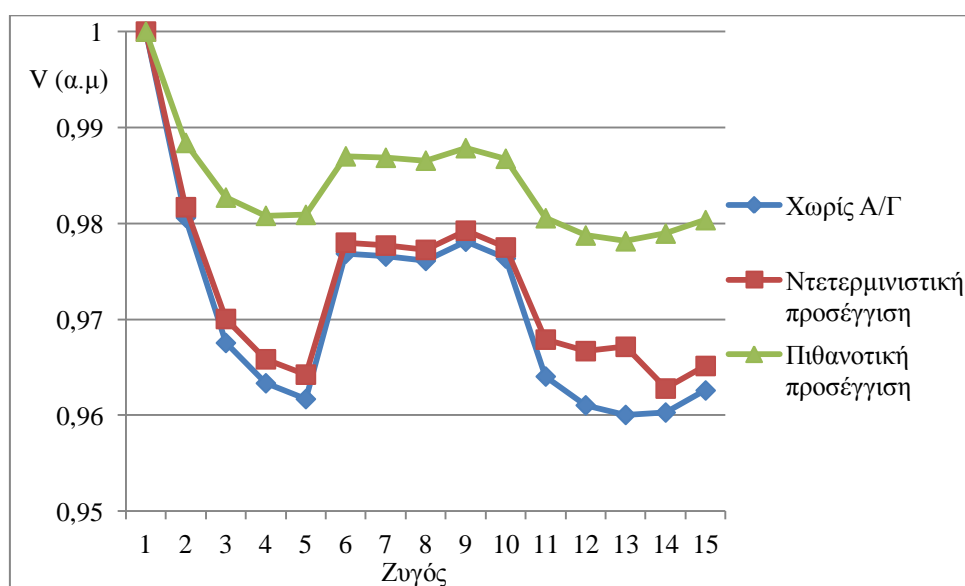
Σχήμα 7.7: Τάση των ζυγών κάθε προσέγγισης για το δικτύου 15 ζυγών.
