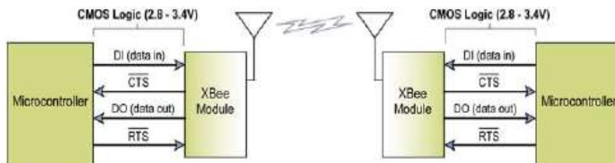
Εικόνα 37: Λογική λειτουργίας της μονάδας XBee module.
