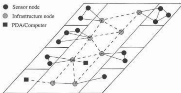
Εικόνα 9: Αρχιτεκτονική Δικτύου εφαρμογής Code Blue.
