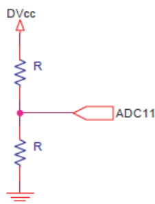
Εικόνα 26: Κύκλωμα μετατροπής σε ενδείξεις τάσης.
