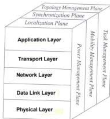
Εικόνα 6: Στοιβά Πρωτοκόλλου Ασύρματων Δικτύων Αισθητήρων.
