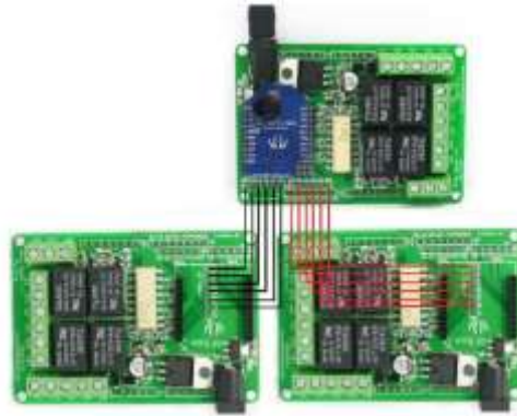
Εικόνα 35: Ένα RFBee ελέγχει τρεις πλακέτες Relay Shield.
