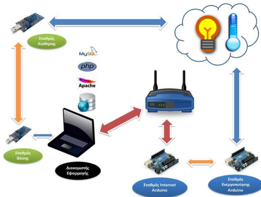
Εικόνα 45: Σχεδιαστική λογική της εφαρμογής ευφυούς οικείας.
