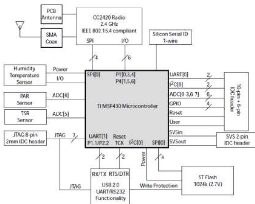
Εικόνα 12: Διάγραμμα μπλοκ συνδέσεων δομοστοιχείων της πλακέτας Tmote Sky με τον μικροελεγκτή.
