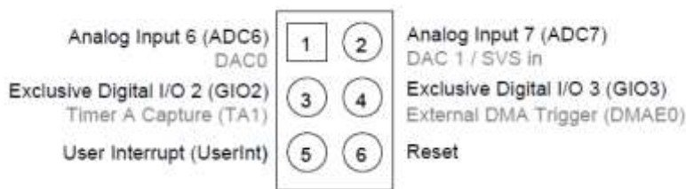
Εικόνα 24: Διάγραμμα ακροδεκτών του Tmote Sky.
