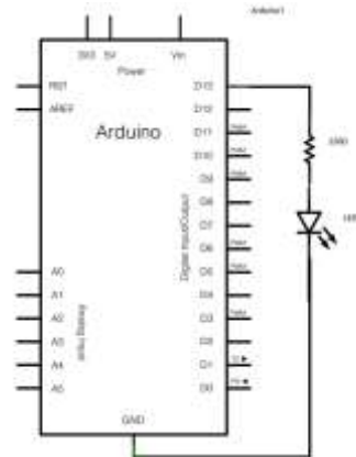
Εικόνα 40: Το κυκλωματικό διάγραμμα της συνδεσμολογίας.
