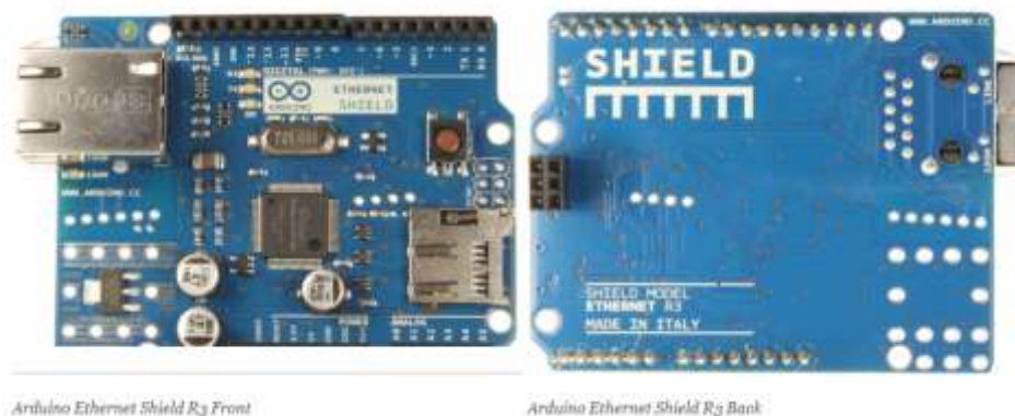
Εικόνα 30: Όψεις πλακέτας Ethernet Shield.
