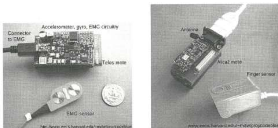
Εικόνα 8: Υλοποιήσεις της εφαρμογής Code Blue με Telos mote και MicaZ mote.
